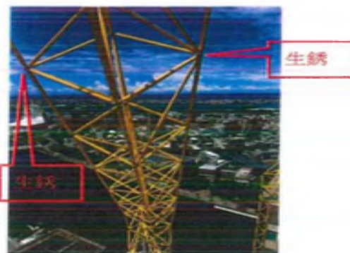
桁架接頭照片(16)
