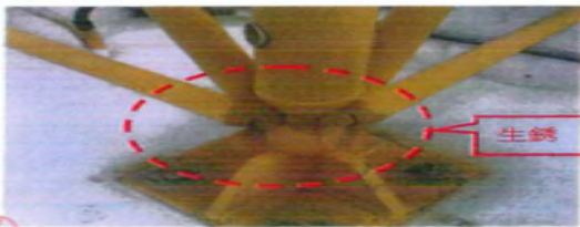
桁架接頭照片(3)
