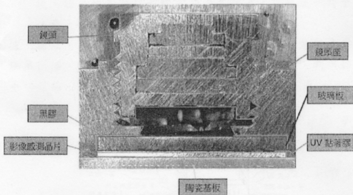
系爭鏡頭模組之實體剖面照片
