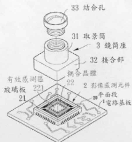
系爭專利第一實施例之立體分解圖
