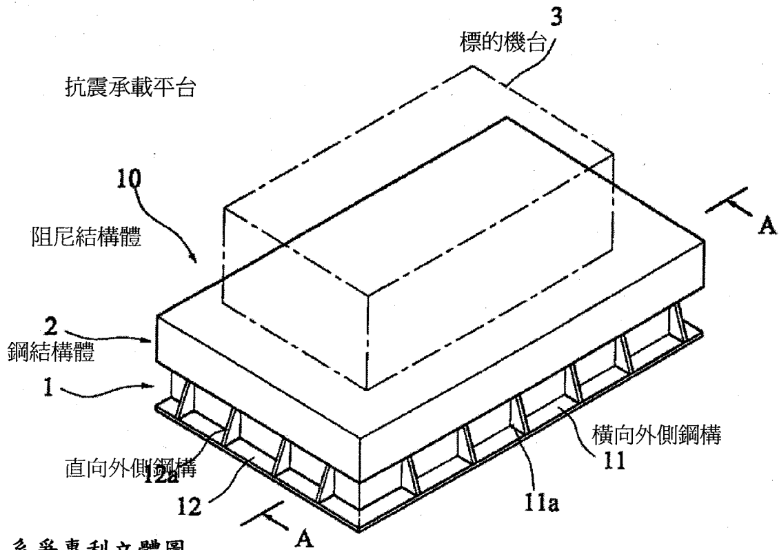
圖 1 系爭專利立體圖
