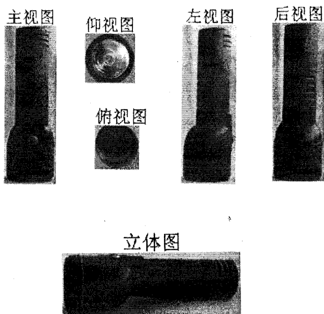
圖示 14(即被證 14, 中國大陸申請號第 97315090.4 號(公告第 CN3102433 號)「斜式手電筒」專利
