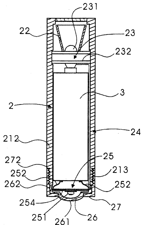
圖示 8(即被證 8，我國第 M303320 號「小型手電筒」新型專利)
