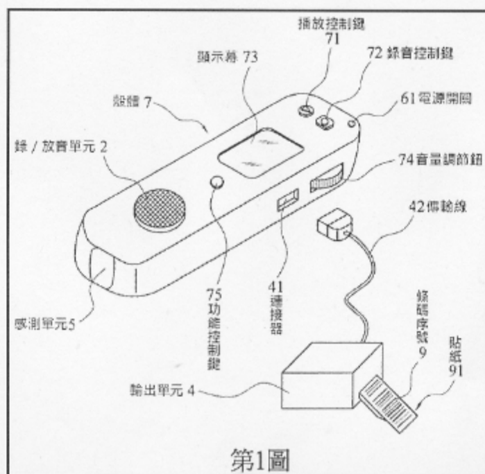
附圖 2：被證 2 第 1 圖為其立體外觀示意圖
