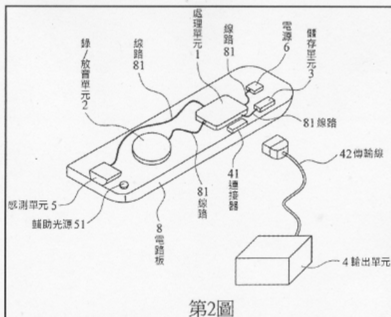
被證 2 第 2 圖為其內部配置之示意圖
