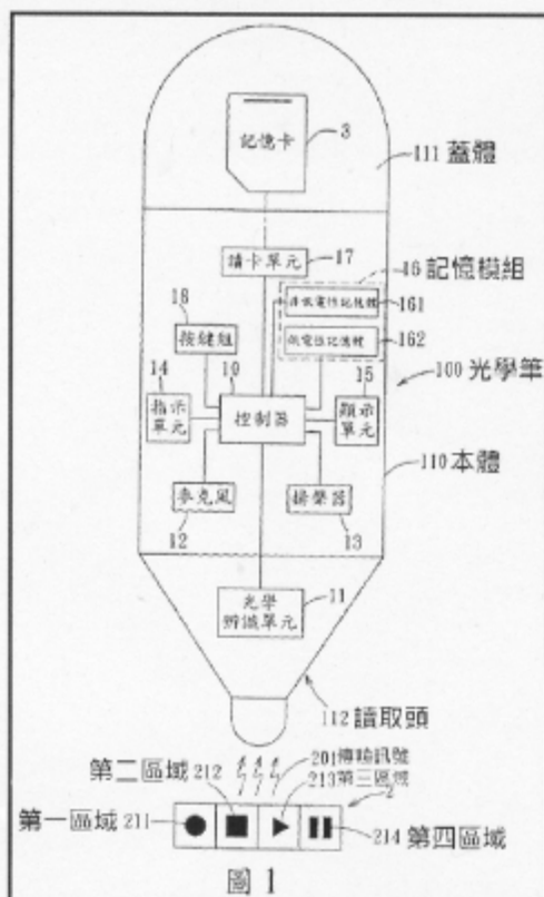
附圖 1：系爭專利圖式一圖 1 為電路方塊圖
