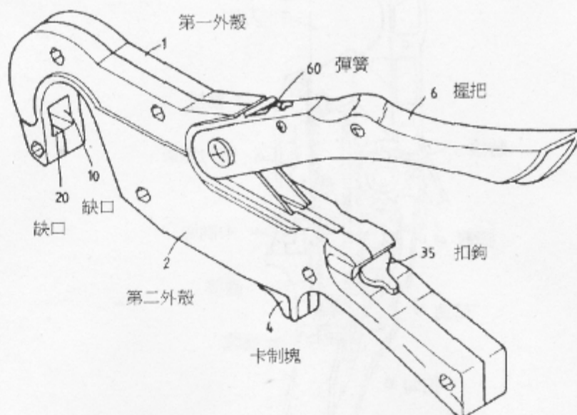
圖示 3-1(即證據 3，86 年 12 月 01 日公告之我國第 321974 號「切管器結構」專利案)
