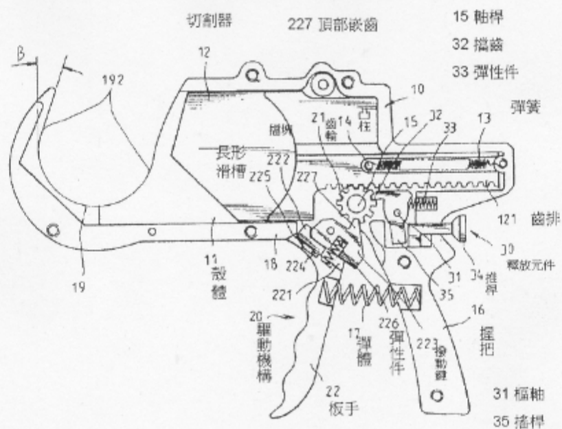
圖示 4(即證據 4, 90 年 12 月 21 日公告之我國第 469920 號「塑膠管專用切割器之改良構造」專利案)
