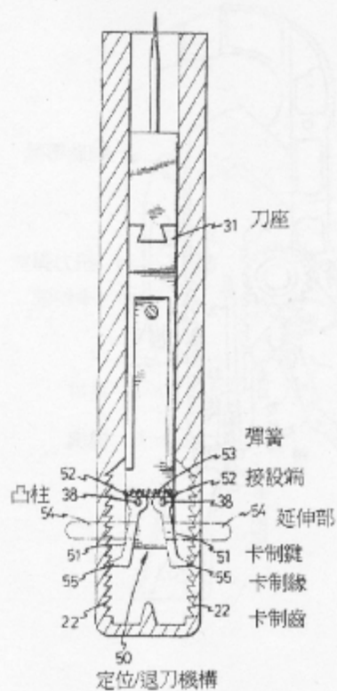
圖示 3-1(即證據 3，86 年 12 月 01 日公告之我國第 321974 號「切管器結構」專利案)
