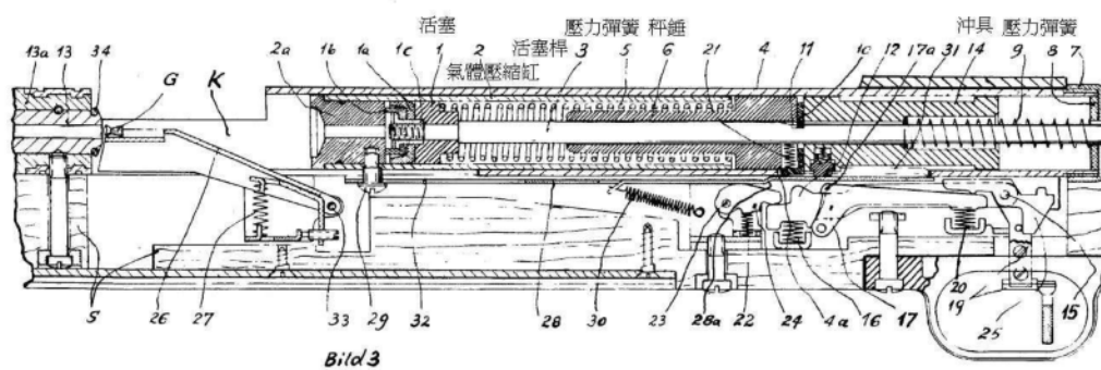
玩具槍裝彈時之縱剖面圖
