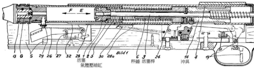
玩具槍發射後縱剖面圖
