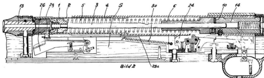
玩具槍發射後縱剖面圖
