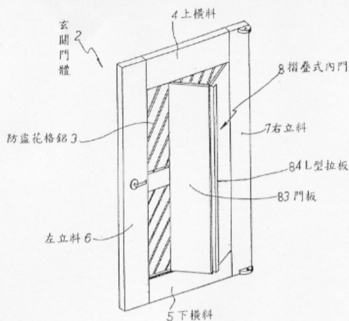
附表四：證據 5 主要圖式
