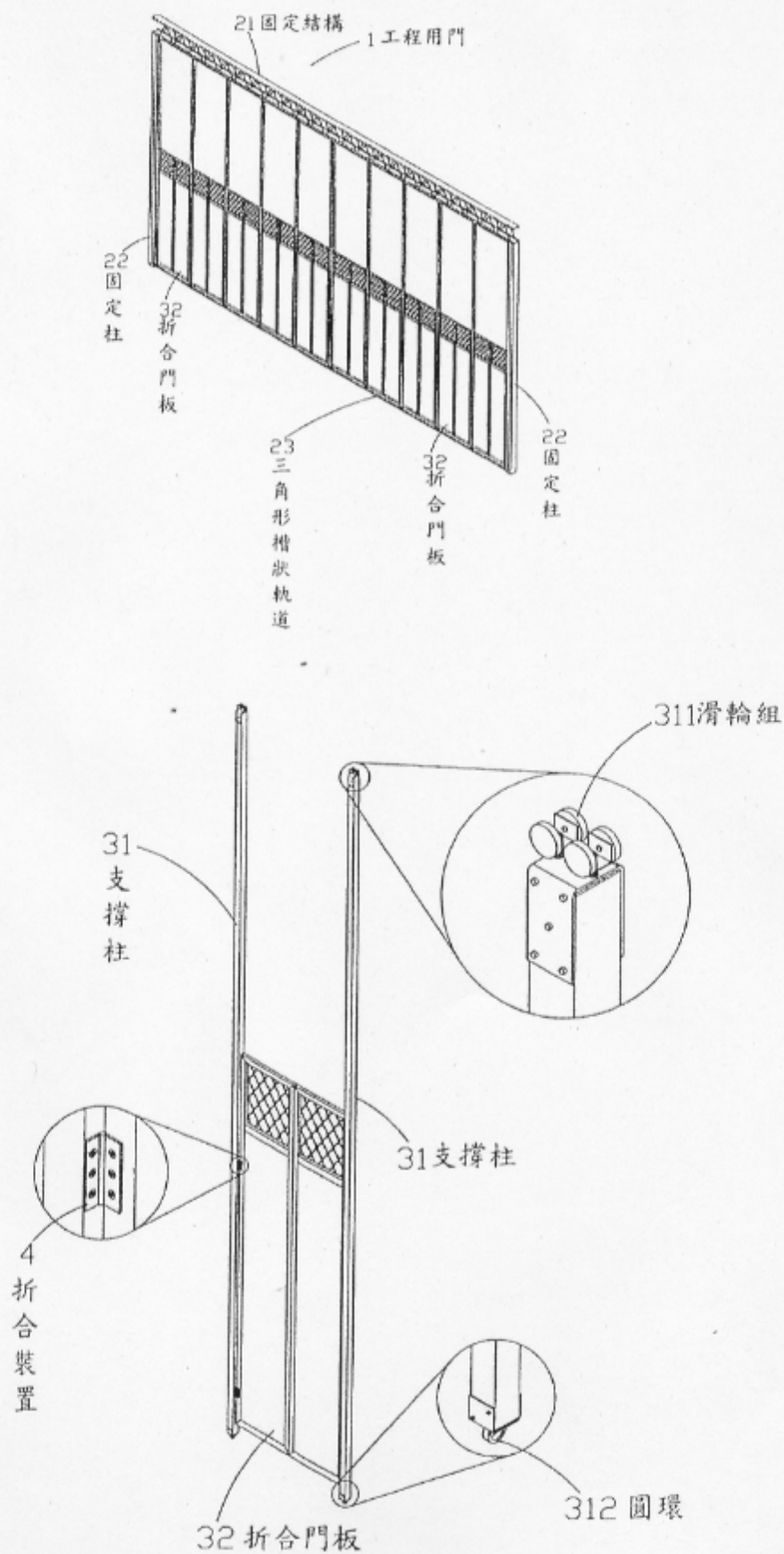
附表一：系爭專利主要圖式
