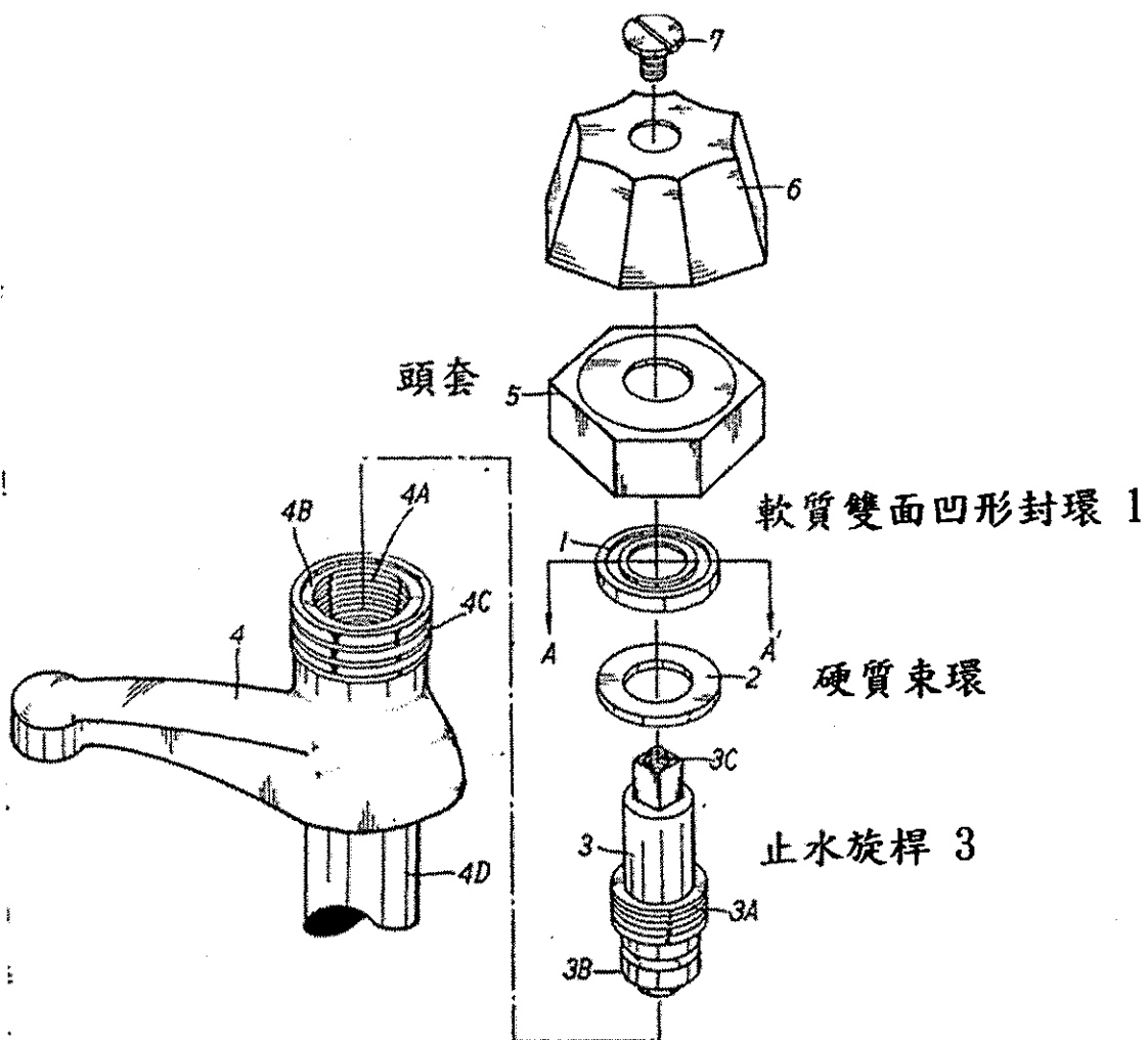
附圖 4：證據五之構件示意圖
