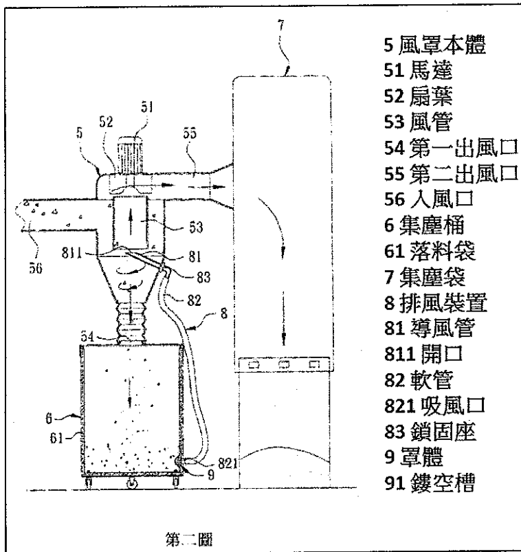
圖示 2-1(即證據 2，為我國申請第 97211845 號「可撐開落料袋之負壓式集塵機」 專利案)
