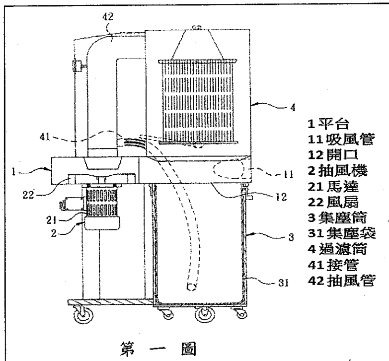
圖示 2-2(即證據 2 說明書所載之先前技術)
