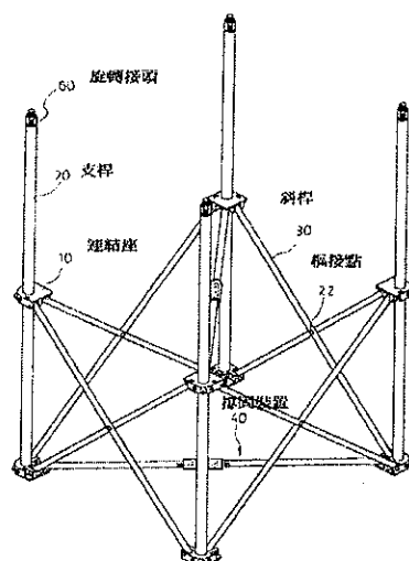
圖示 1-1(即參加人系爭專利)
