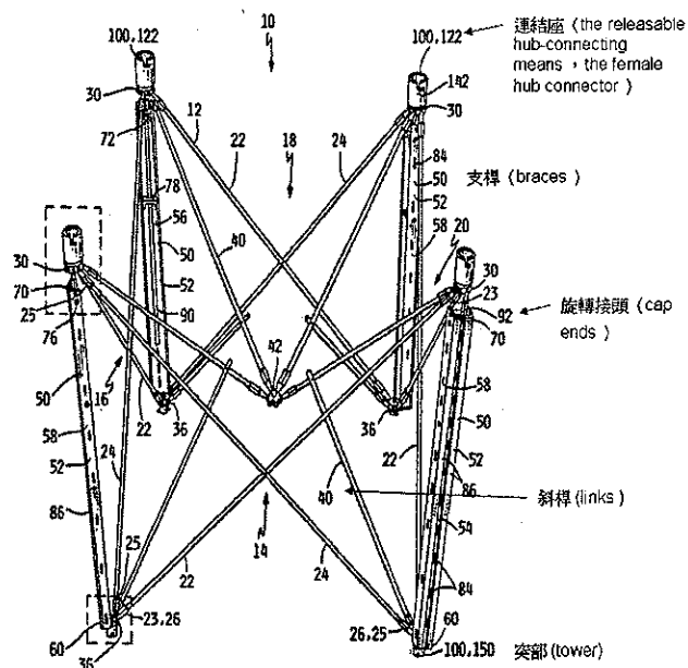
圖示 2-1(即證據 2，係 1994 年 7 月 12 日公告之美國第 5327700 號「Collapsible Modular Display Tower Assembly」專利案)
