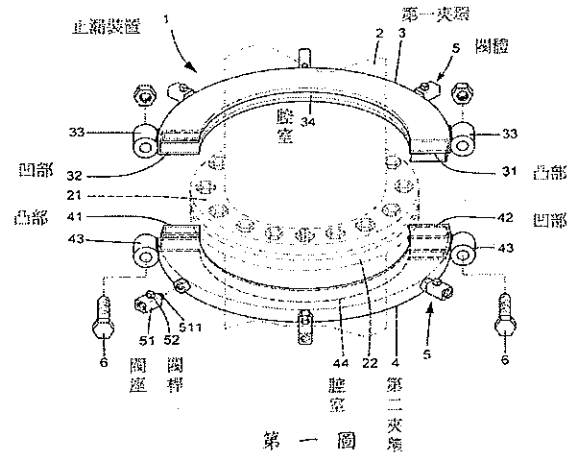
附表一：系爭專利主要圖式
