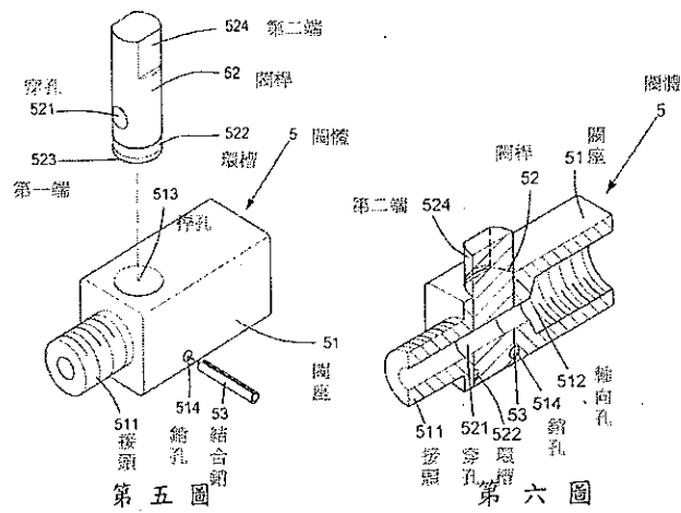
附表二：證據二主要圖式
