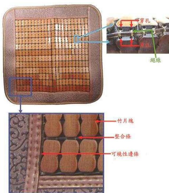
《圖一：待鑑定物之正面視圖》
