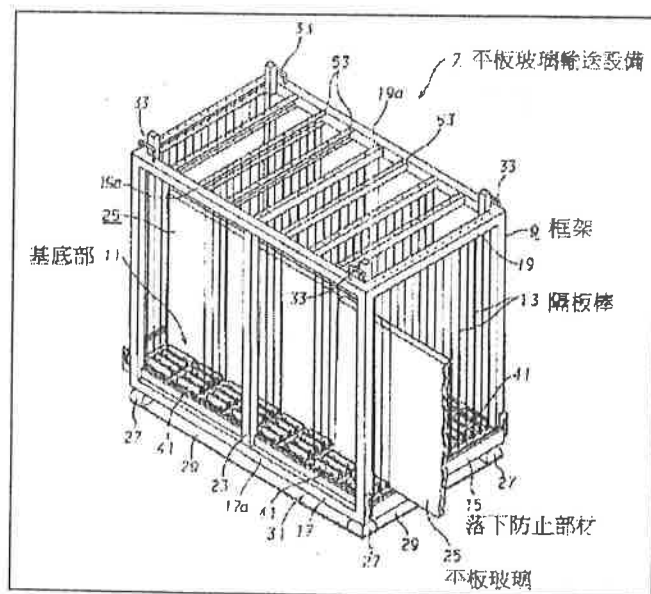
被證 4 圖 1 揭露平板玻璃輸送設備之示意圖
