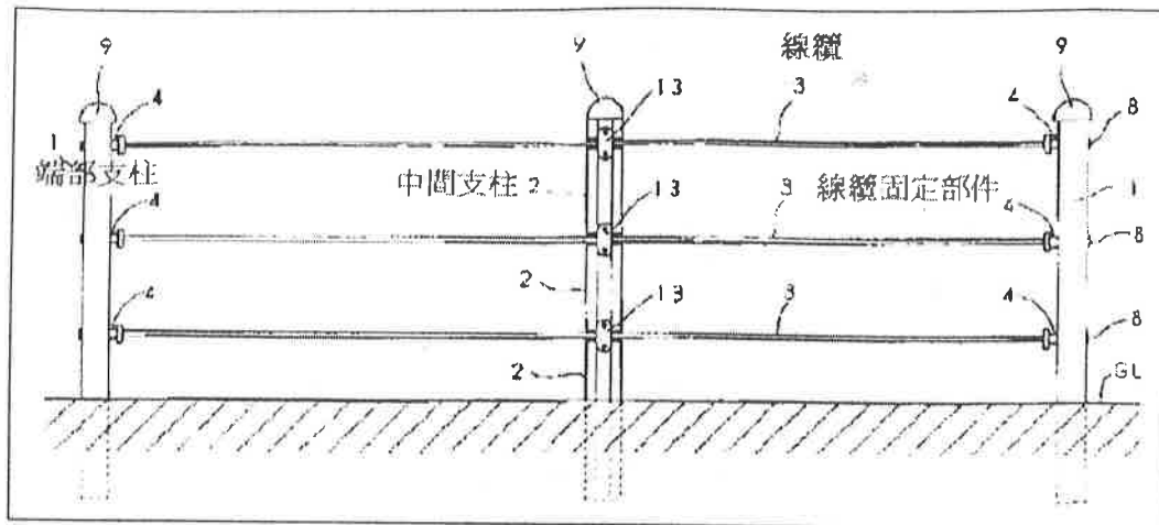
被證 3 圖 1 揭露張設型線纜式柵欄之示意圖
