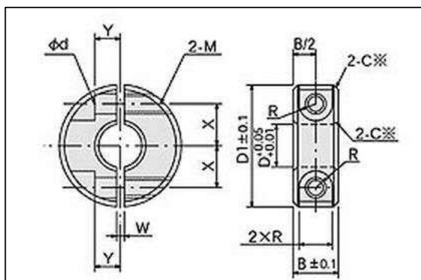
メカ工業(株)之「固定環」設計圖 (參原證 27 號上側)
