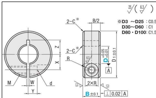
原告之「固定環」設計圖 (參原證 15 號第 2 頁)
