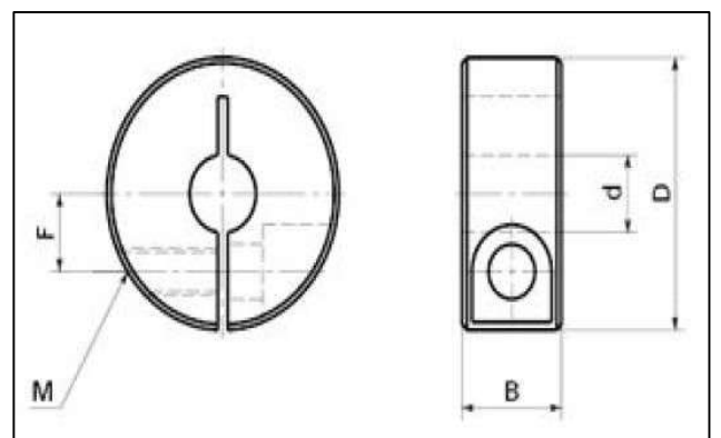
鍋屋バイテック会社之「固定環」 設計圖 (參原證 28 號上側)
