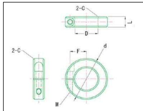
小西製作所之「固定環」設計圖 (參原證 25 號左側)
