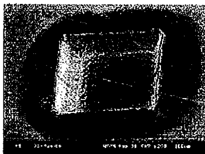
圖 5-7 空氣中加工 50 層
