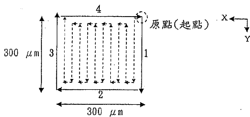
圖 5-3 正方形切層加工路徑
