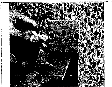
五、待鑑定對象之迫緊單元拆卸示意圖(一):
