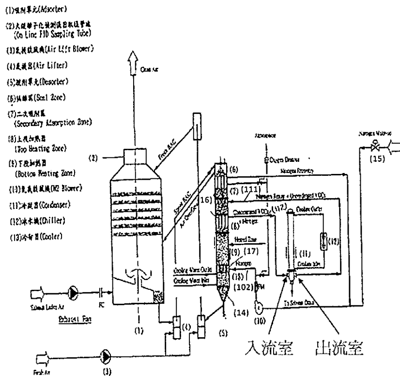
圖3-1 活性炭流體化床系統流程圖
