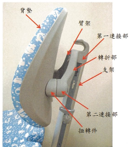
背墊未受力
