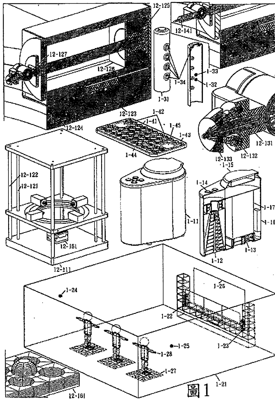
系爭新型專利圖 1：即時互動 3D 立體仿製娛樂裝置示意圖
