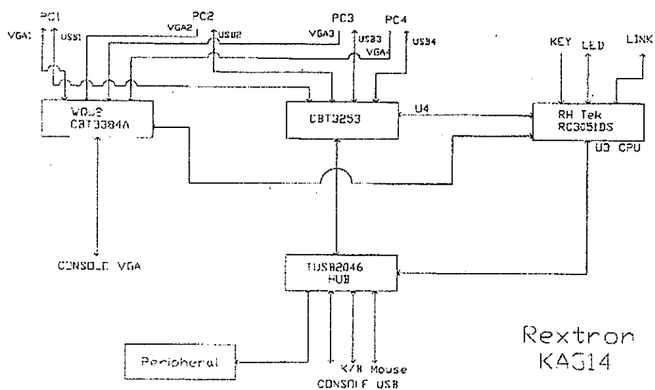
KAG14 電路圖
