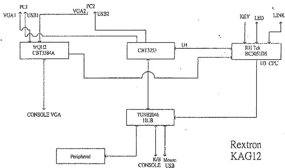
KAG12 電路圖
