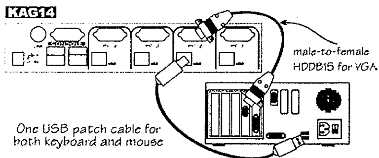
KAG14 之電腦連接示意圖
