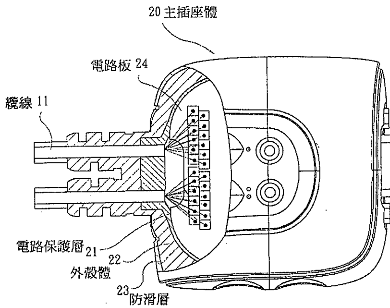
系爭新型專利第五圖：主插座體之局部剖示圖
