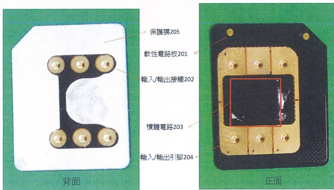
系爭產品2-2(micro-SIM貼片卡200)
