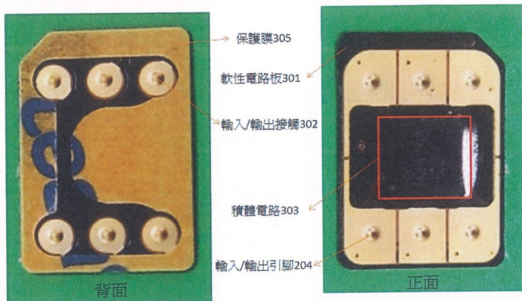
系爭產品2-3(nano-SIM貼片卡300)
