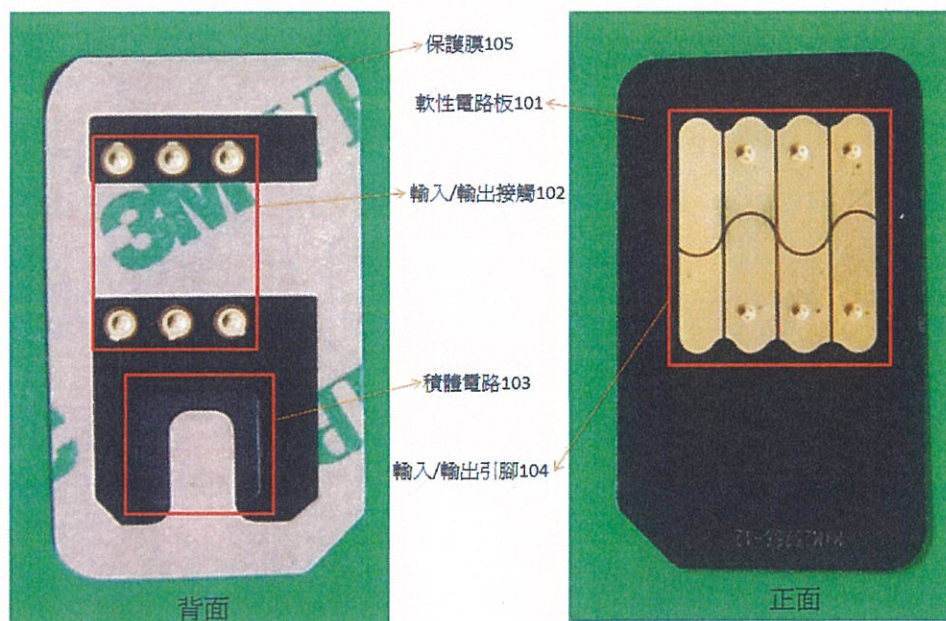
系爭產品2-1(mini-SIM貼片卡100)
