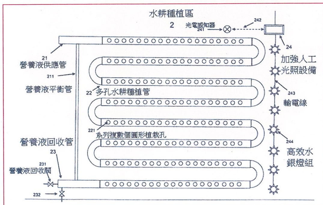
第三圖為系爭專利之水耕種植區系統配置圖
