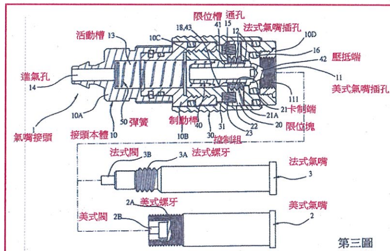
系爭專利第三圖組合剖面圖
