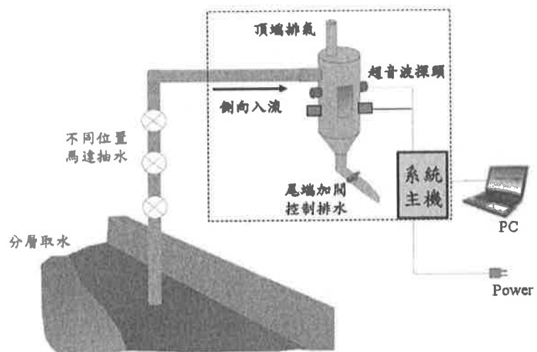
圖(一) 抽取式超音波泥砂濃度量測系統
