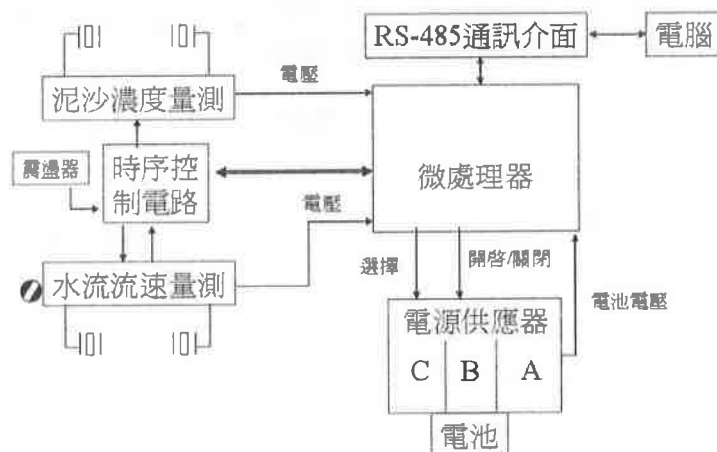
圖 5-1 系統整體功能方塊圖
