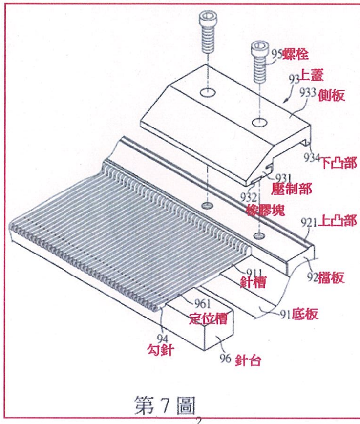
系爭專利第7圖係習用針織機夾針組之立體外觀圖
