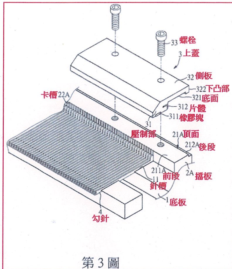
系爭專利第3圖係第二實施例之立體外觀圖
