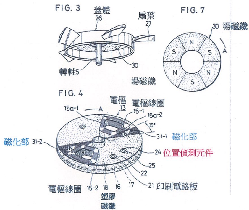
圖 3、4、7 單相無刷馬達之結構
