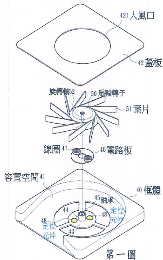
圖 1 薄型散熱構造之立體分解示意圖
