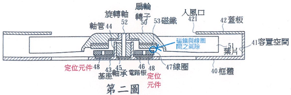
圖 2 薄型散熱構造剖面圖
