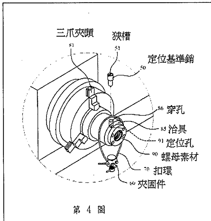
第 4 圖為滾珠螺母結構之第二裝配加工示意圖
