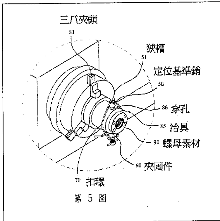
第 5 圖為滾珠螺母結構之第三裝配加工示意圖
