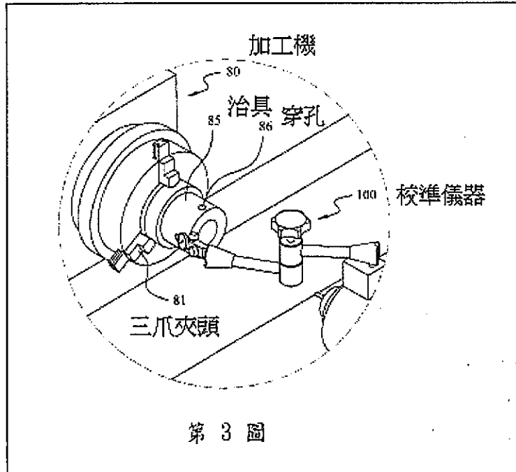
第 3 圖為滾珠螺母結構之第一裝配加工示意圖
