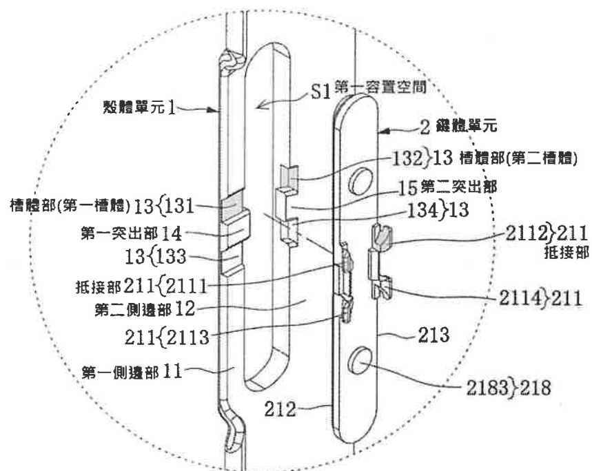
2.圖 2C 為圖 2A 之 A 部分之局部放大分解示意圖
