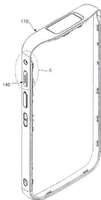
1.圖 1 為移動終端之終端本體立體圖
