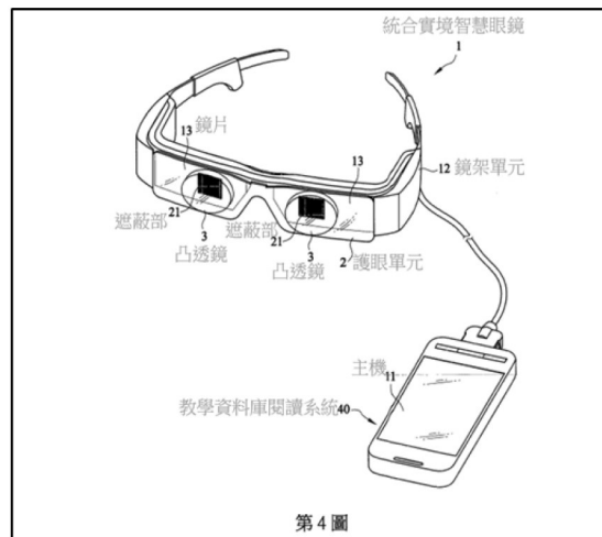
圖 4 為具有凸透鏡之立體組合圖
