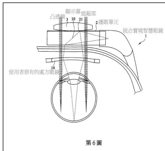
圖 6 為應用時之效果示意圖
