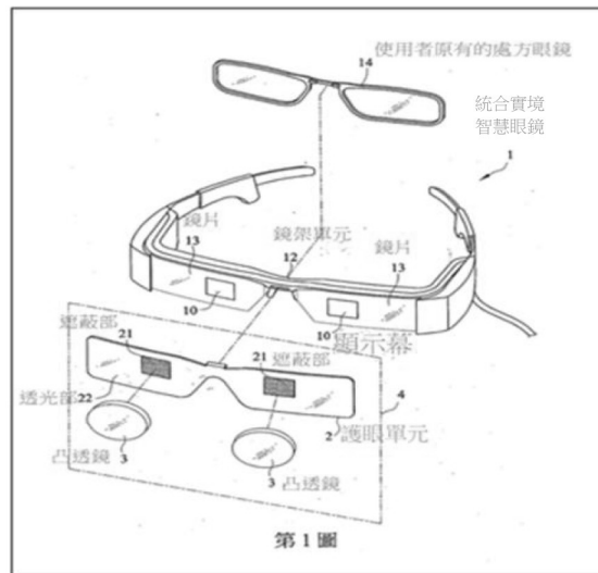
圖 1 為立體分解圖
