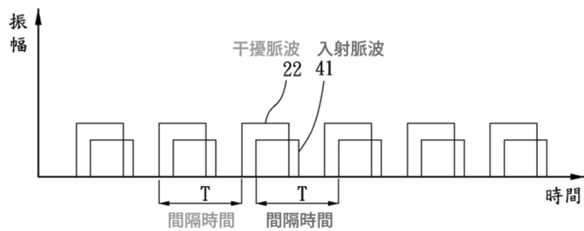
系爭專利圖 6 為訊號干擾示意圖
