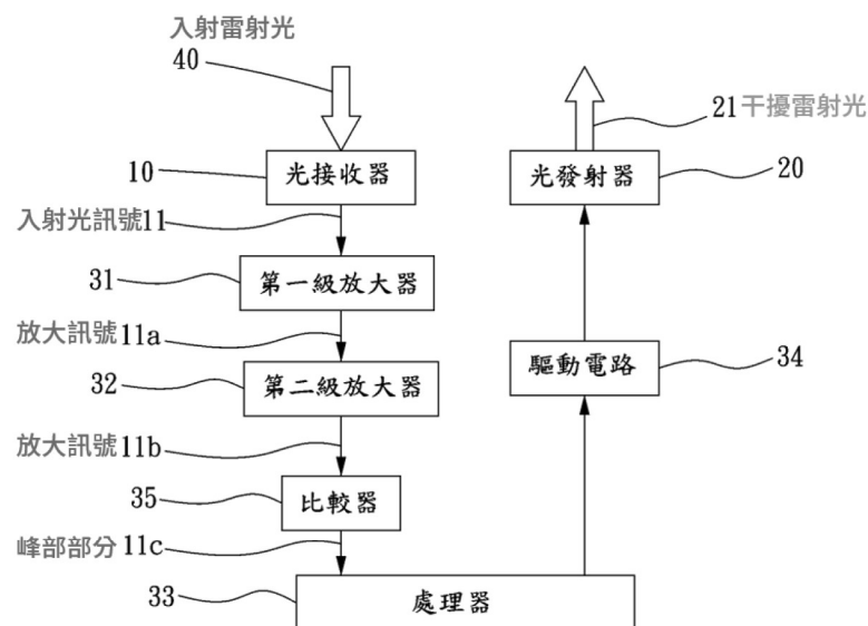
系爭專利圖 4 為雷射干擾器之結構關係方塊圖
