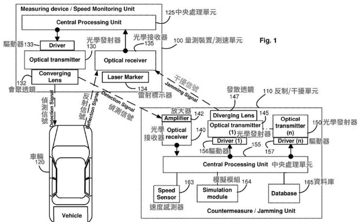
甲證 4 圖 1 為測速單元與反制/干擾單元之示意圖
