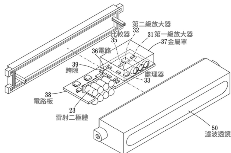
系爭專利圖 2 為雷射干擾器之分解圖
