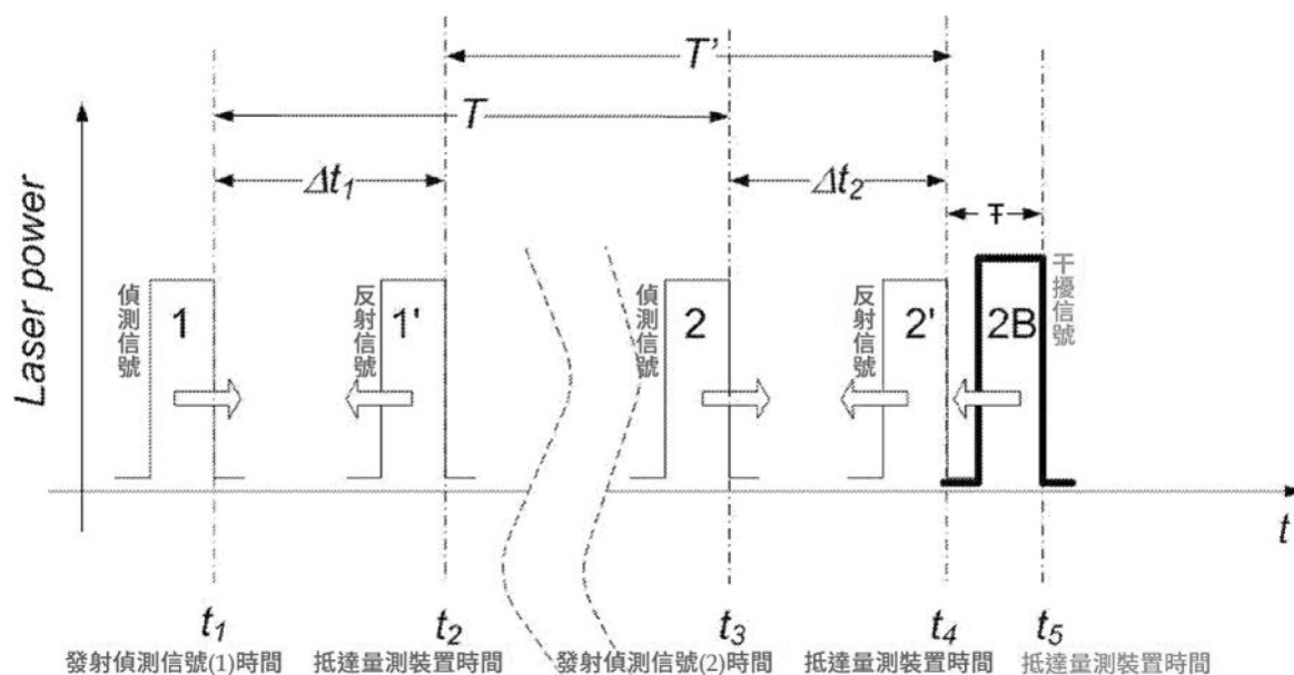
甲證 4 圖 3 為偵測信號與干擾信號之時域圖
