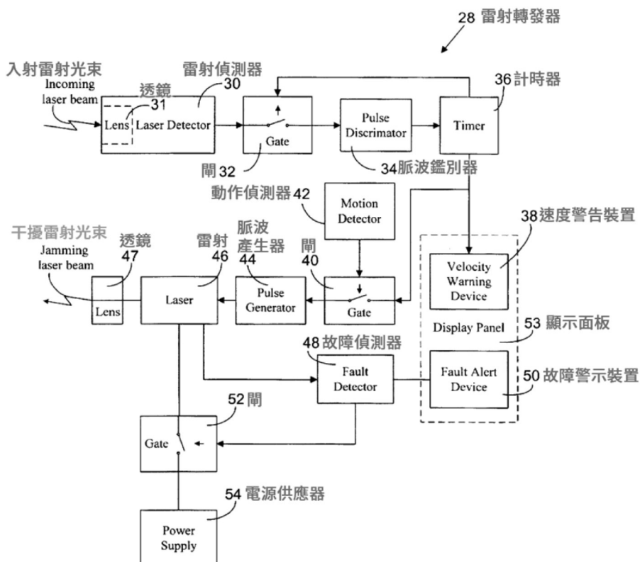
甲證 1 圖 4 係雷射轉發器之方塊圖
