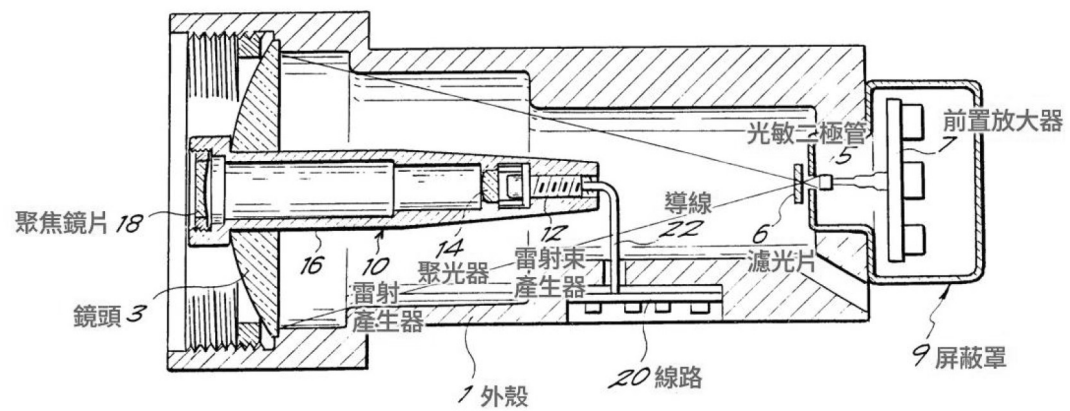
甲證 6 圖 1 係為雷射產生器和接收器的剖面圖
