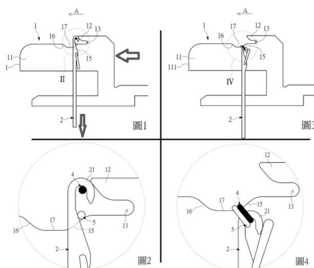
圖 1 至 4 為申克片沿前進方向 A，第一推紗面 15 推動第二紗線示意圖
