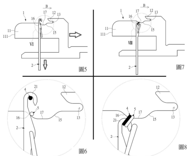
圖 5 至 8 為申克片沿後退方向 B，第二推紗面 16 推動第二紗線示意圖
