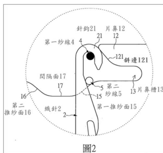
圖 2 為圖 1 的 II 部分詳圖
