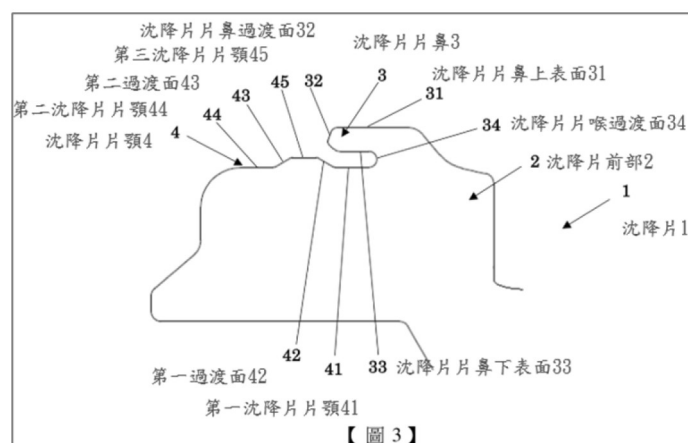
圖 3 為沈降片的放大側視圖
