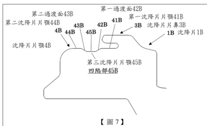
圖 7 為實施例 3 的沈降片的放大側視圖
