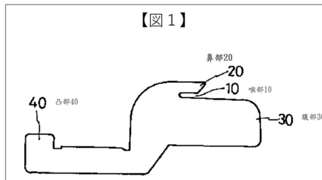
圖 1 為傳統織布機中所使用的沉降片的側面圖
