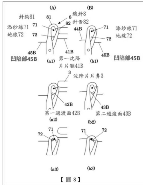
圖 8 為實施例 3 的沉降片的在(A)第一軌道及(B)第二軌道上的織針下降時的針鉤內的線之位置的概略圖
