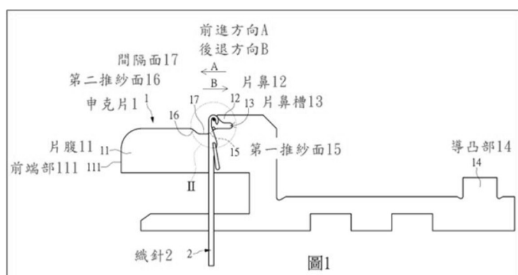
圖 1 為單面互調雙色提花圓編結構的動作示意圖
