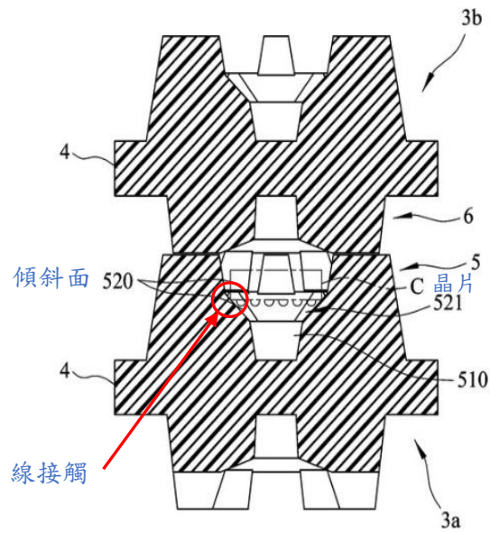
[圖 10]為證據 3 圖 6 一晶片置於該等晶片承載裝置內的剖面圖
