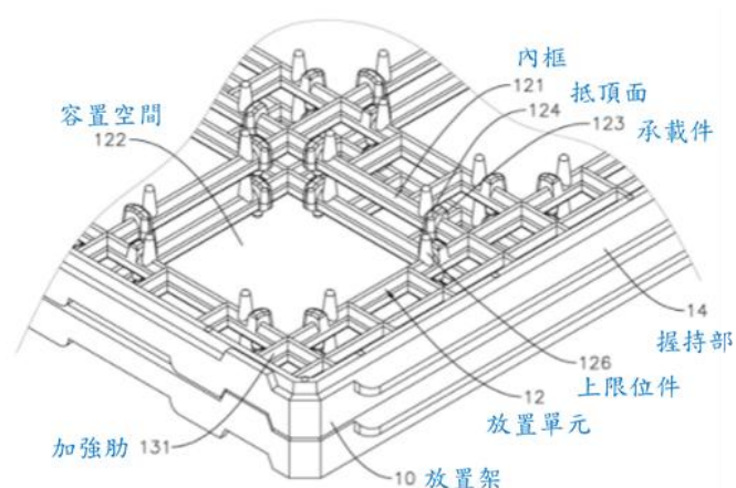
[圖 1]為系爭專利圖 3 局部放大圖
