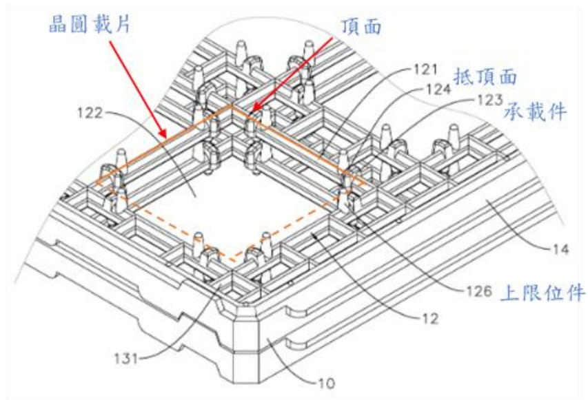
[圖 7]為系爭專利圖 3 清洗治具局部放大圖
