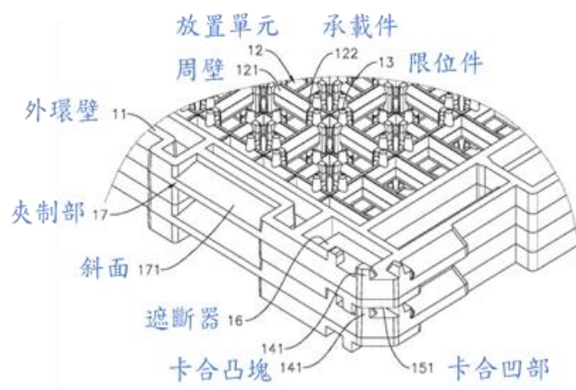
[圖 3]為證據 2 圖 3 放置架角落的立體圖
