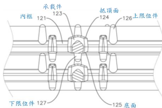
[圖 2]為系爭專利圖 4 局部剖面圖
