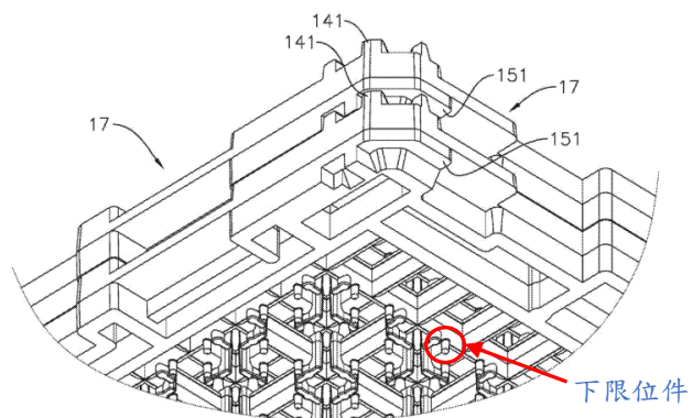
[圖 10]為證據 3 圖 6 一晶片置於該等晶片承載裝置內的剖面圖
