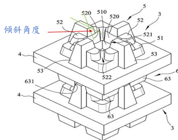
[圖 9]為證據 3 圖 4 兩個上下疊置晶片承載裝置之立體圖
