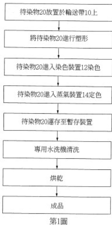
第 1 圖 自動化混合染色製程方塊示意圖
