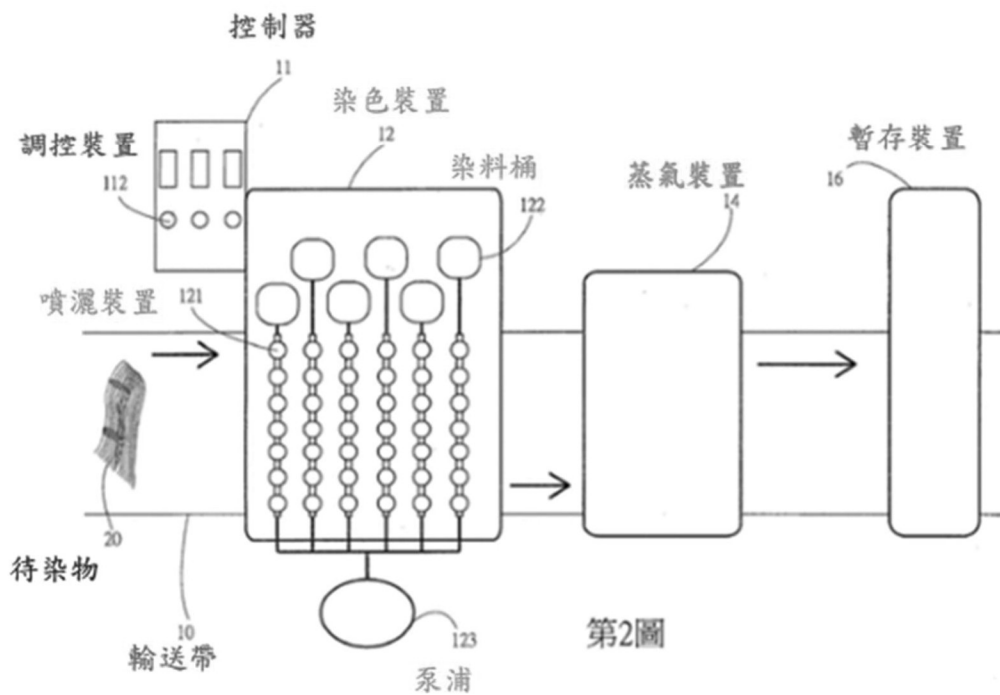
第 2 圖 系統示意圖
