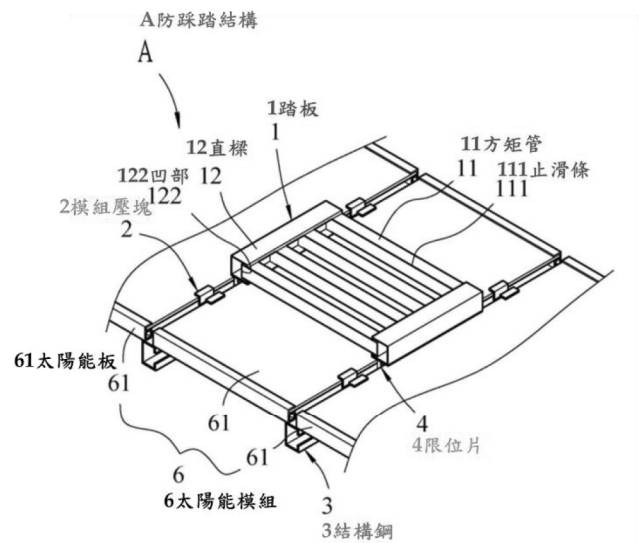
圖 1 太陽能板防踩踏結構之立體外觀圖。
