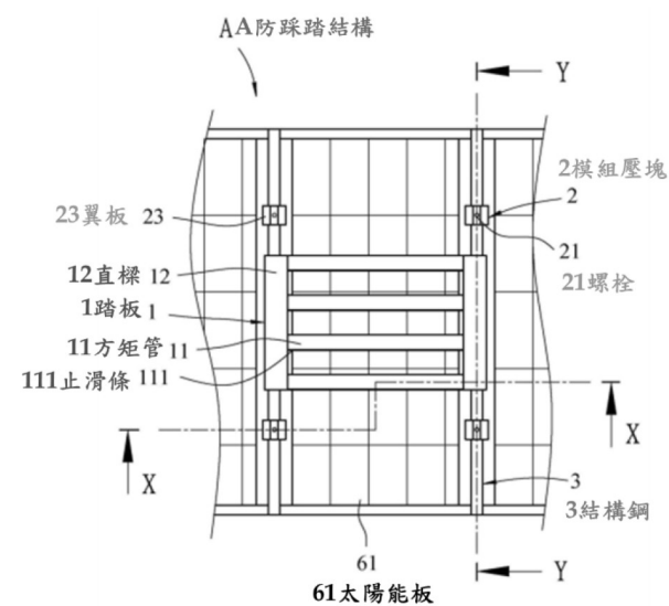
圖 2 太陽能板防踩踏結構之平面圖。
