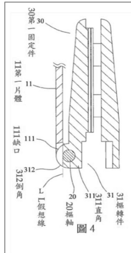
圖 4 為系爭專利第一片體、樞軸、第一固定件之局部剖視圖
