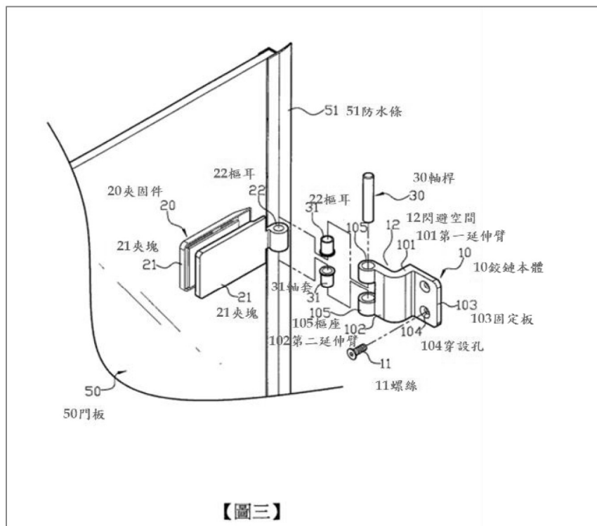
圖三為本創作之立體分解圖
