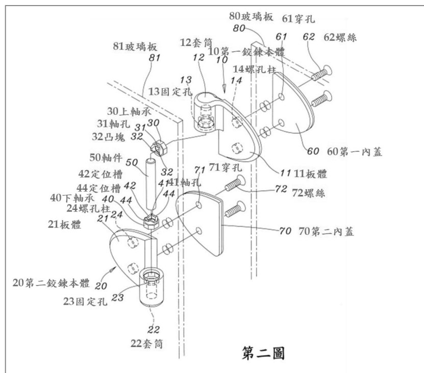
第二圖為本創作之立體分解圖
