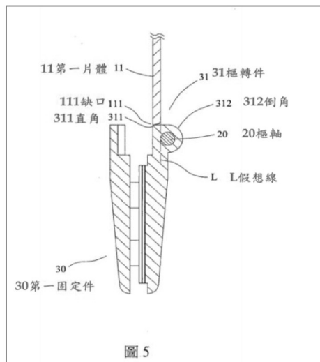
圖 5 為系爭專利第一片體、樞軸、第一固定件之局部剖視圖
