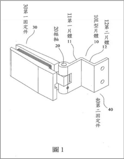
圖 1 為系爭專利一種實施例之外觀示意圖
