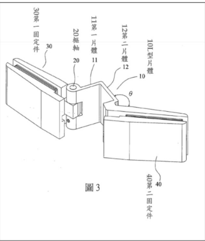
圖 3 為系爭專利再一種實施例之外觀示意圖
