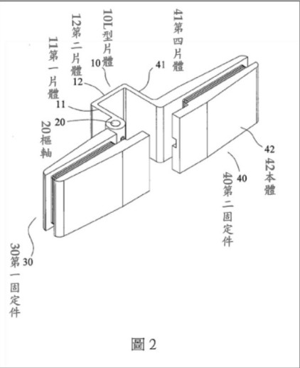
圖 2 為系爭專利另一種實施例之外觀示意圖
