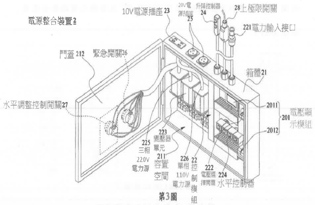
第 3 圖 系爭專利之結構圖
