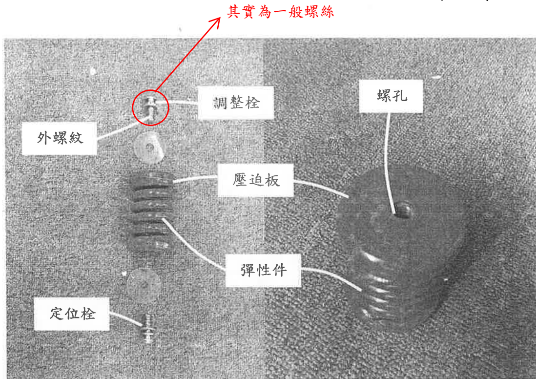
【照片五】— 待鑑定對象之部分元件
