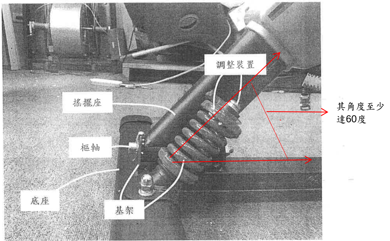
【照片二】、待鑑定對象之立體圖(二)
