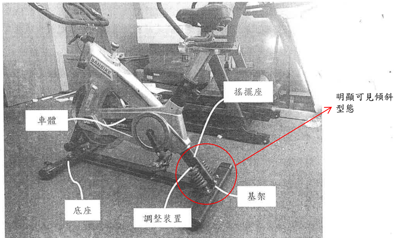
【照片一】、待鑑定對象之健身車整體 (本附圖為原告所提出及標示，紅色字體部分則為本判決所加)
