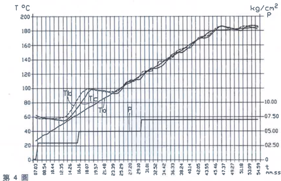
圖 4 系爭專利系統之溫度壓力函數的時間進度圖鎮
