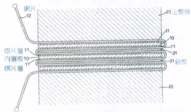
圖 1 熱壓示意圖
