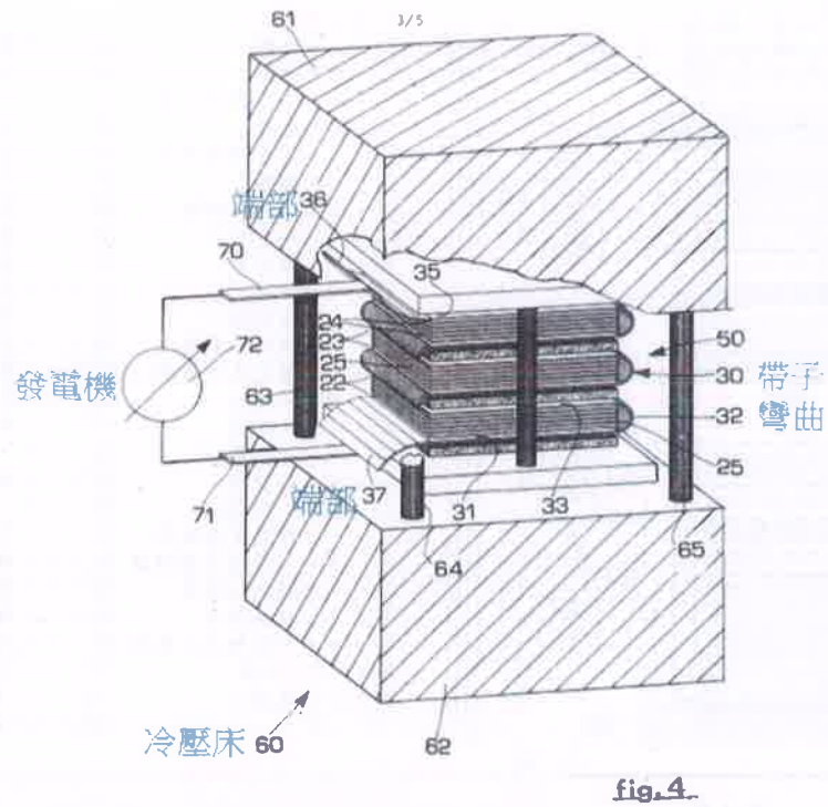
圖 4 生產具金屬薄片之塑膠層板之裝置
