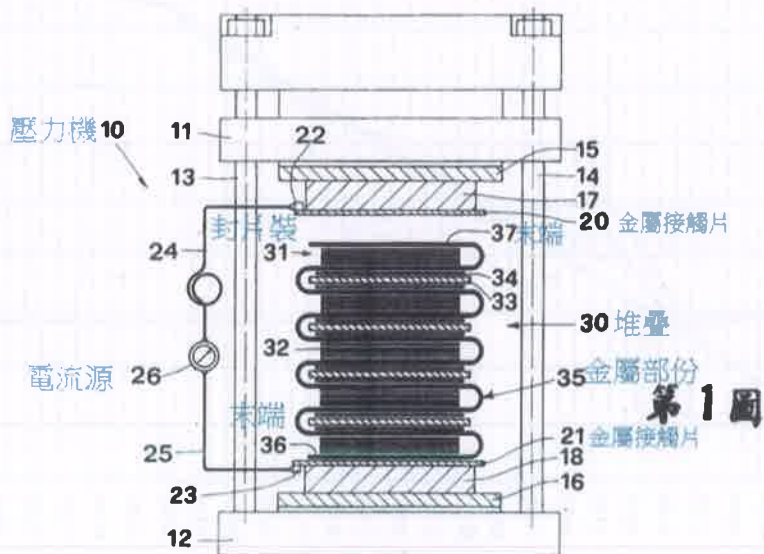
圖 1 製造塑膠層板之壓力機
