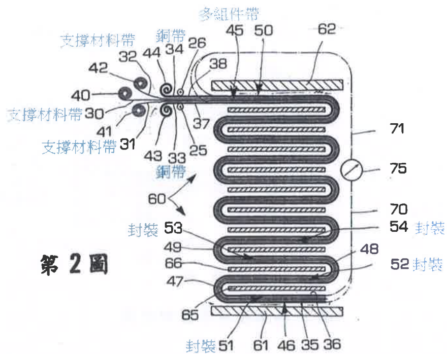
圖 2 製造具有金屬層薄片之塑膠疊層板之加工方法之示意圖
