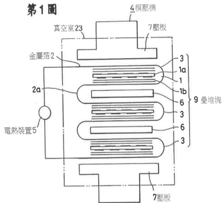
圖 1 積層板製造設備
