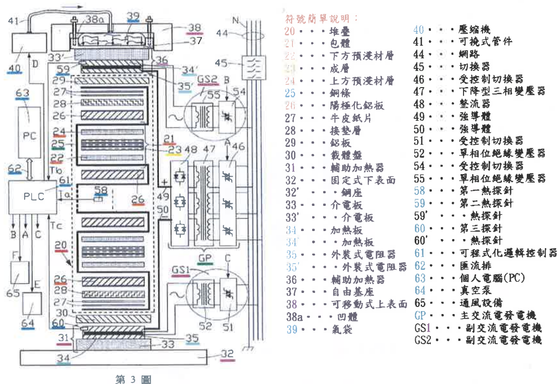
圖 3 系爭專利系統示意圖
