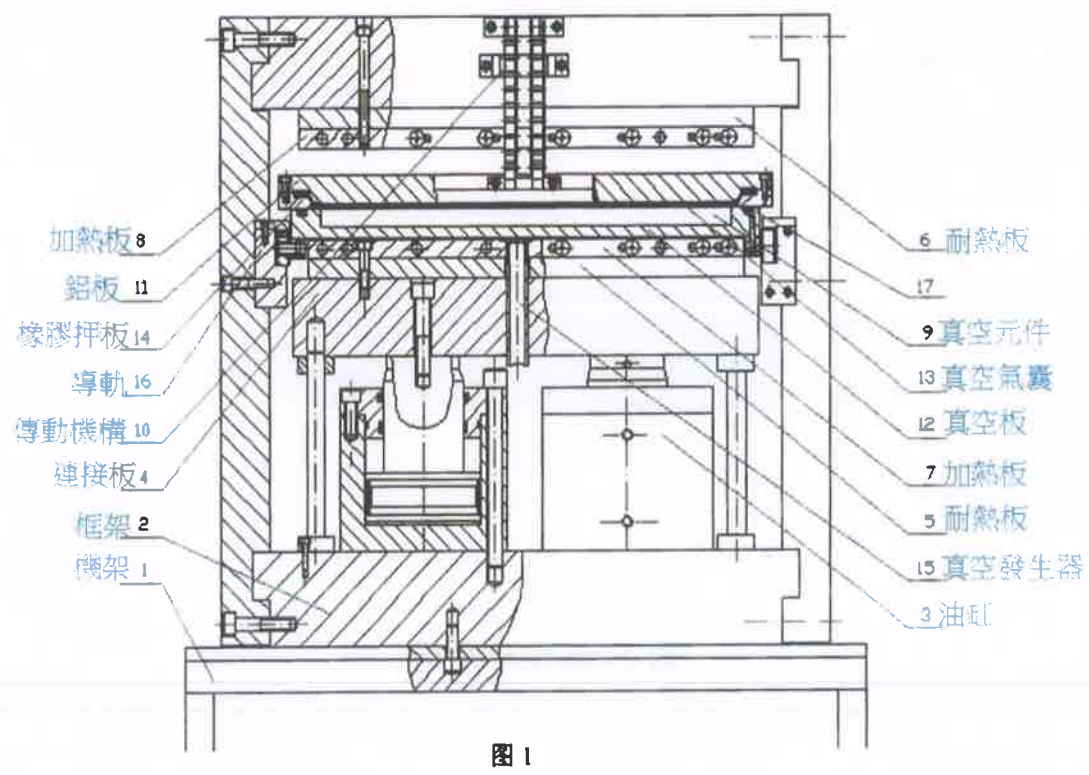
圖 1 軟性線路板真空壓合機
