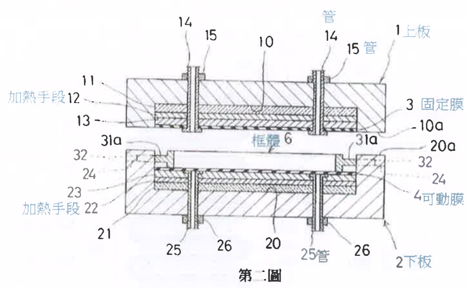
圖 1 真空積層裝置剖視圖
