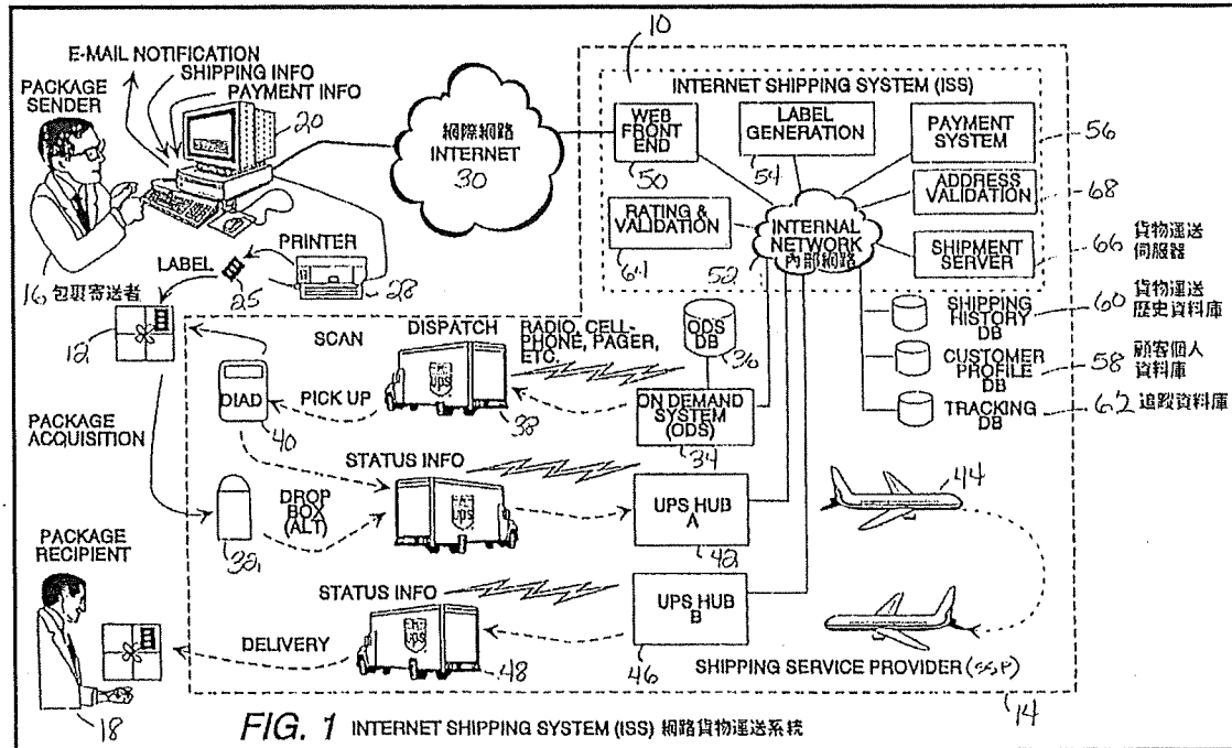
圖 1 為網路貨物運送系統 (Internet Shipping System, ISS) 的架構圖
