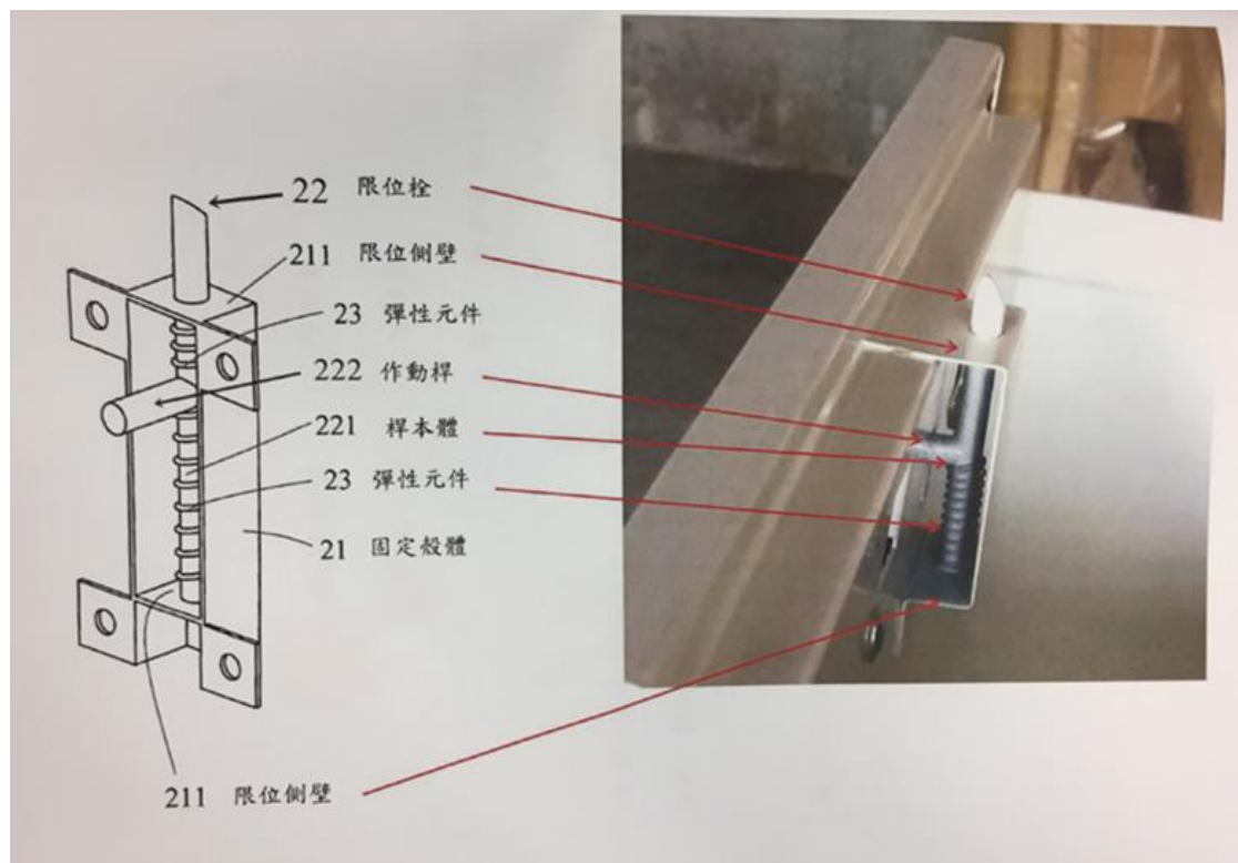
附圖二：系爭產品實物照片
