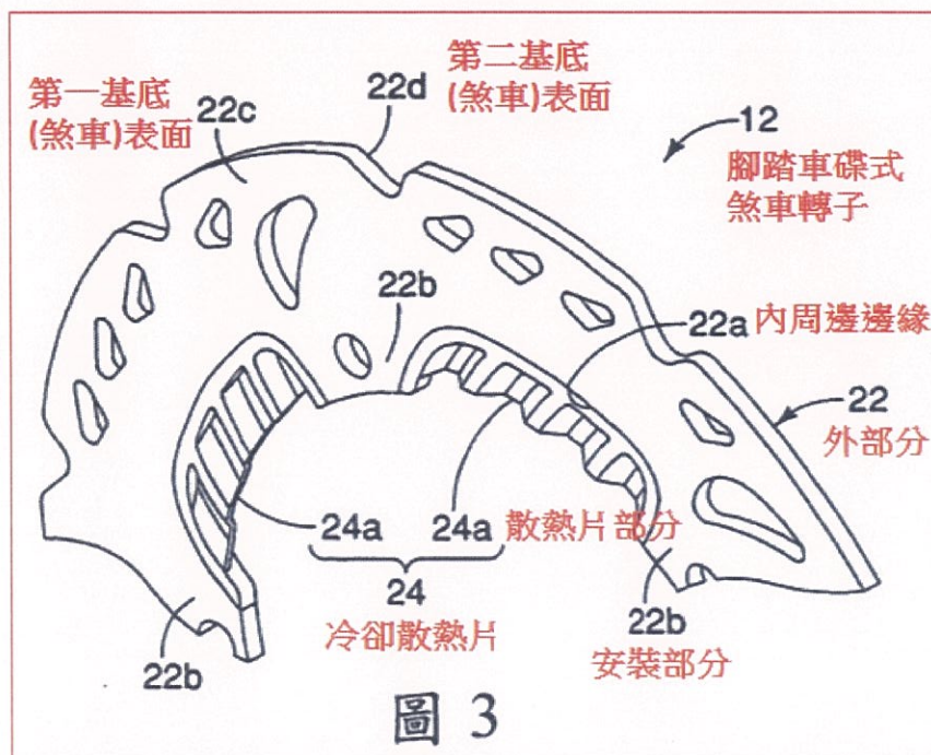
附圖 2：圖 3 係腳踏車碟式煞車轉子之一放大透視圖
