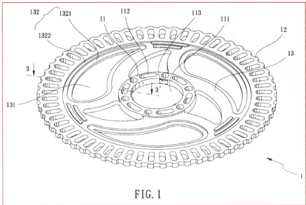
附圖 7：圖 1 係增強盤式製動器轉子之盤式轉子的透視圖
