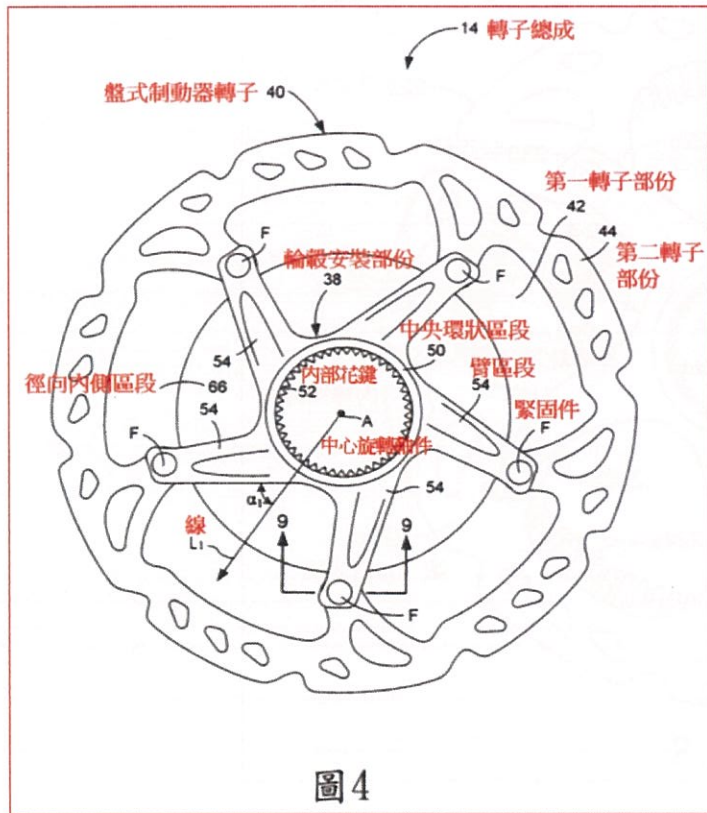
附圖 6：圖 4 為以從自行車移去的方式顯示的盤式制動器轉子的側視圖
