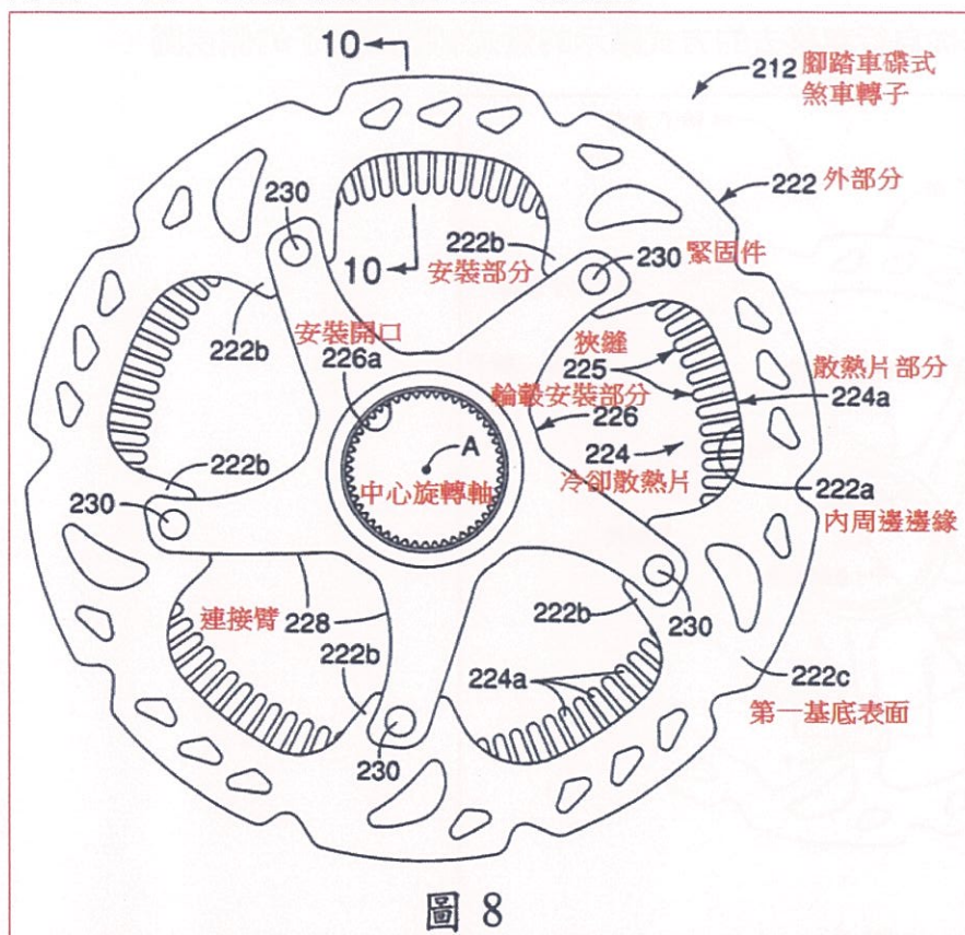
附圖 4：圖 8 係碟式煞車轉子之一側視圖
