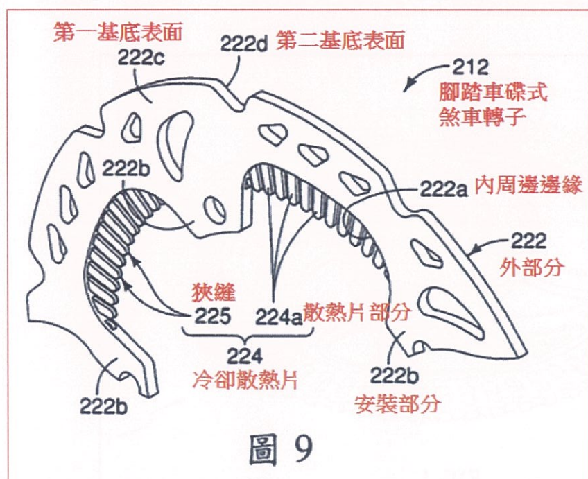
附圖 5：圖 9 係腳踏車碟式煞車轉子之一放大透視圖
