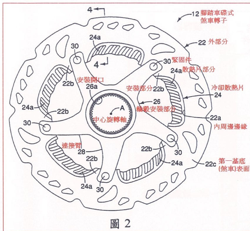
附圖 1：圖 2 係碟式煞車轉子之一側視圖
