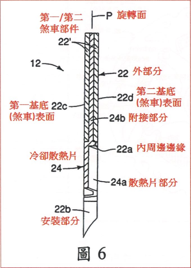
附圖 3：圖 6 係腳踏車碟式煞車轉子之一橫截面圖
