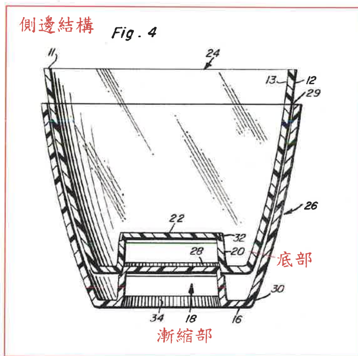
2：圖 4 杯體側視圖
