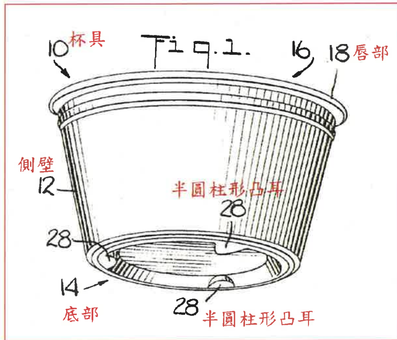
1：圖 1 杯具結構
