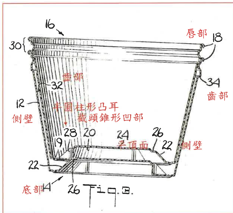
2：圖 3 杯具堆疊結構
