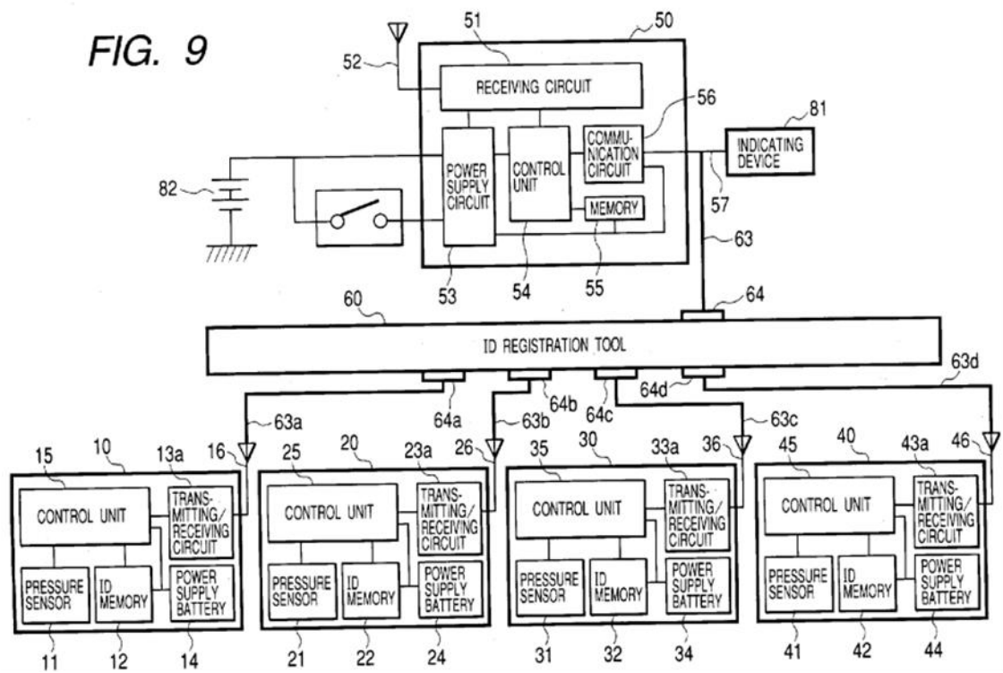
本發明第二實施例之胎壓偵測器之ID註冊裝置的方塊圖
