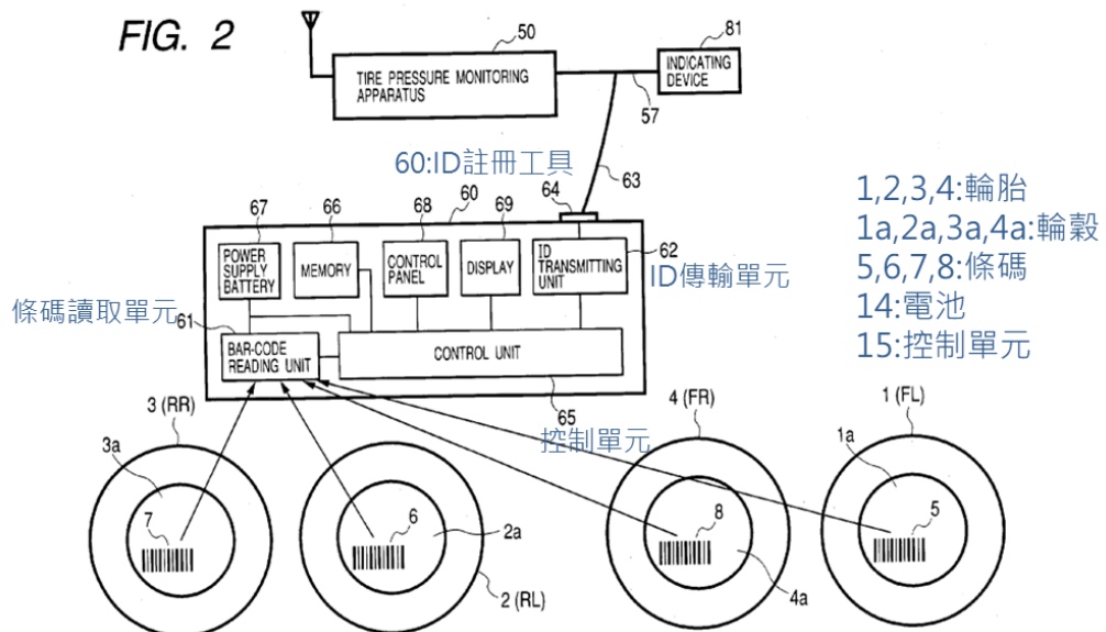
本發明第一實施例之胎壓偵測器之ID註冊裝置的方塊圖
