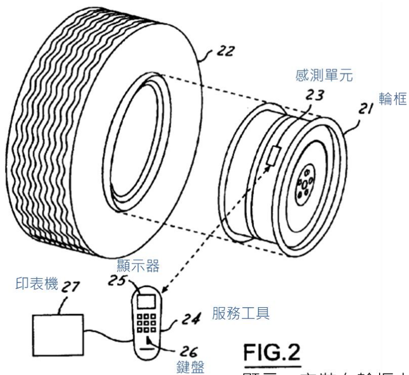
顯示一安裝在輪框上且可與服務工具進行通訊之胎壓偵測單元
