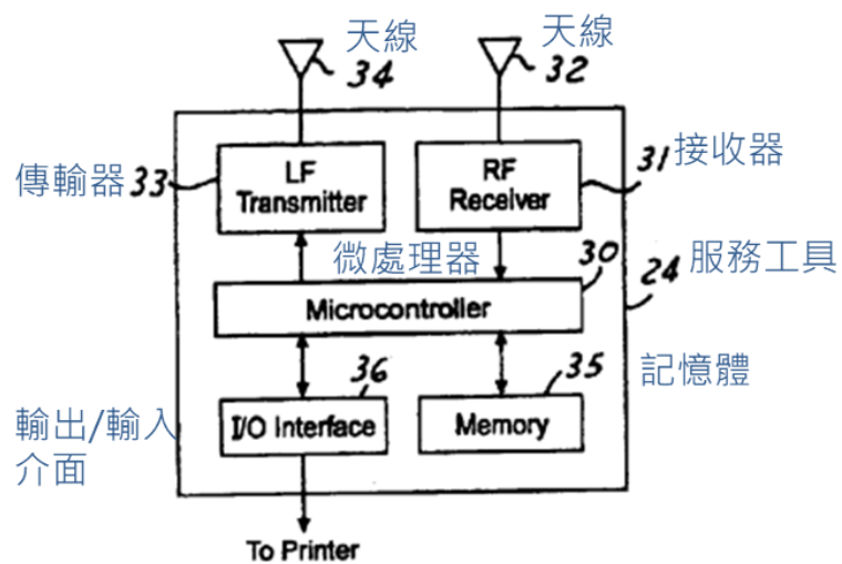
FIG.3 服務工具之細部示意圖
