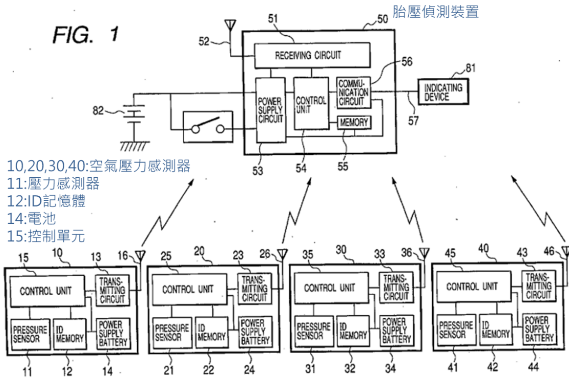
本發明第一實施例之胎壓偵測器之方塊圖
