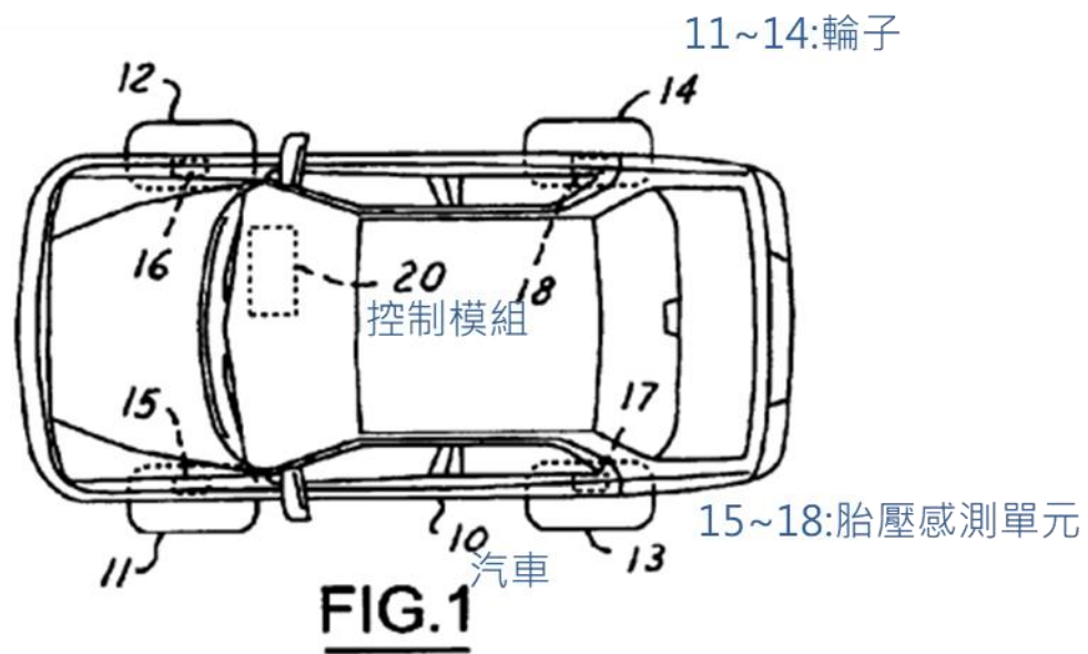
具有胎壓偵測系統之汽車
