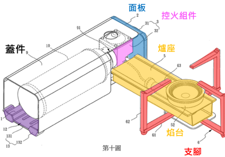
7. 第十圖：系爭專利各支腳的另一實施例立體示意圖
