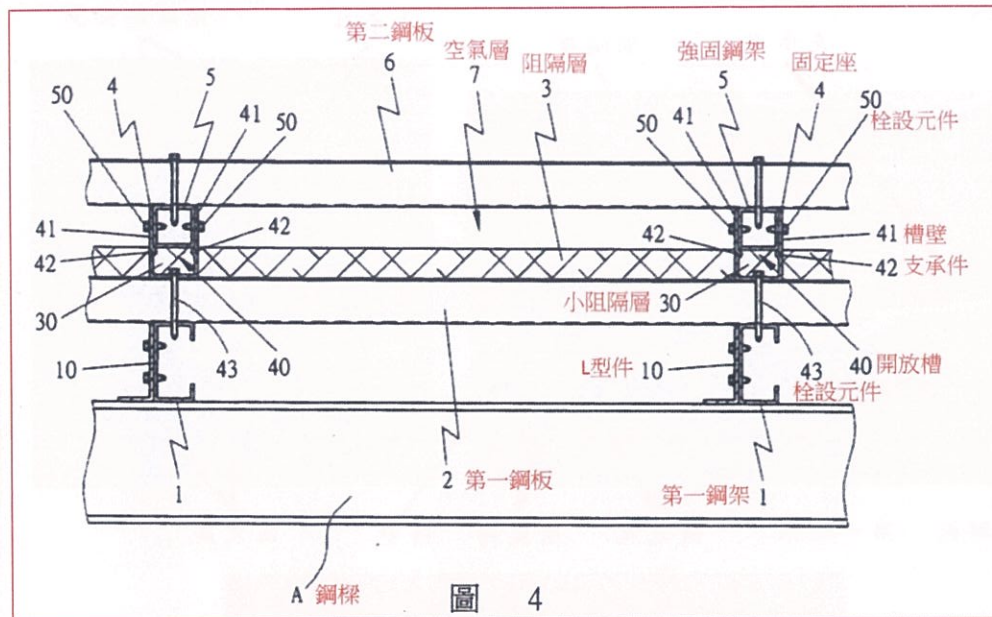
第 4 圖為複合鋼板實施例之前視圖
