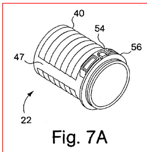
圖 7A 為帶載體的立體圖
