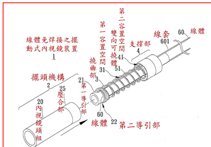
第 2 圖為線體免焊接之擺動式內視鏡裝置一視角之組合示意圖
