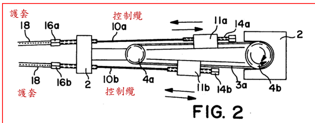
圖 2 為圖 1 切線方向側視圖，其有一對控制線之機構
