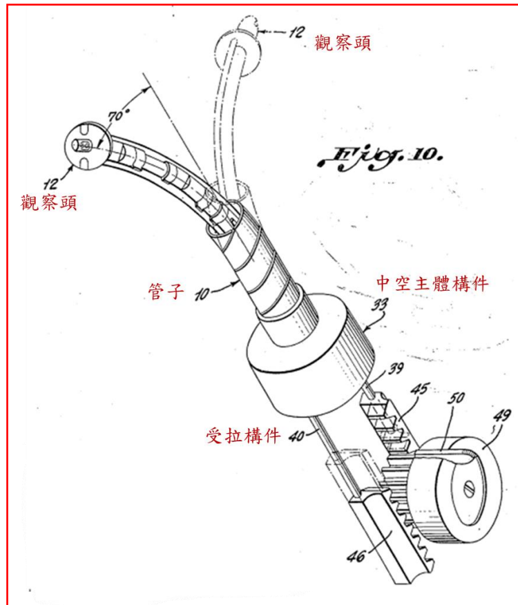
圖 10 為胃鏡管彎曲機構之透視放大圖
