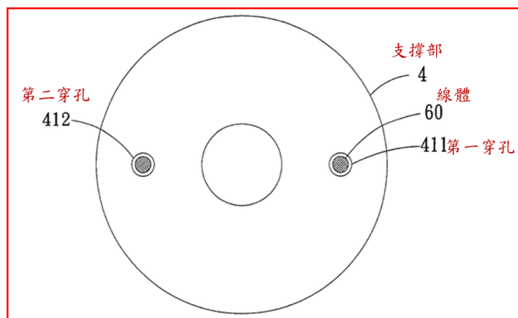
第 3 圖為擺動式內視鏡裝置之支撐部底部之一視角示意圖
