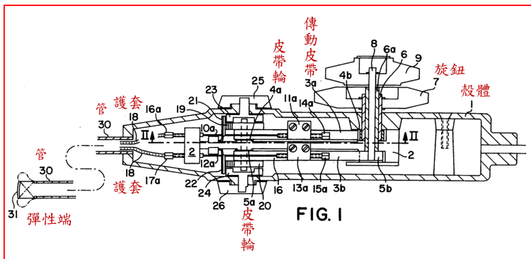
圖 1 為操縱器元件橫截面的側視圖
