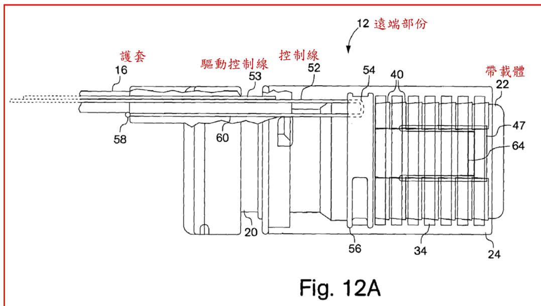
圖 12A 為遠端部分之局部截面側視圖
