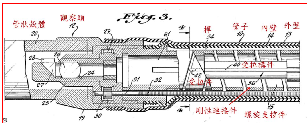
圖 3 為胃鏡管彎曲機構之剖視放大圖
