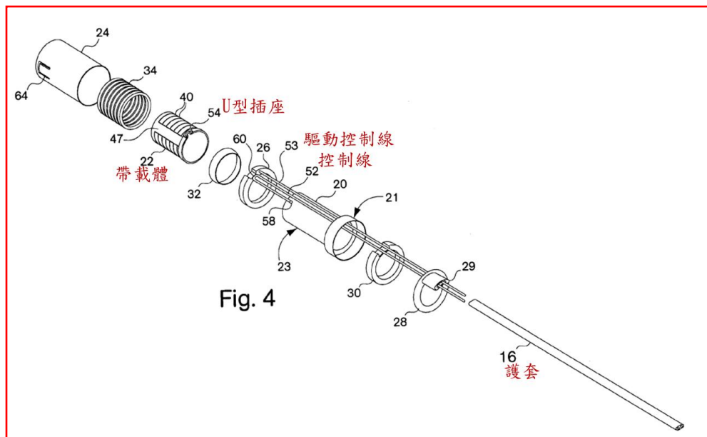
圖 4 為內窺鏡分配器的遠端部分之部件分解圖
