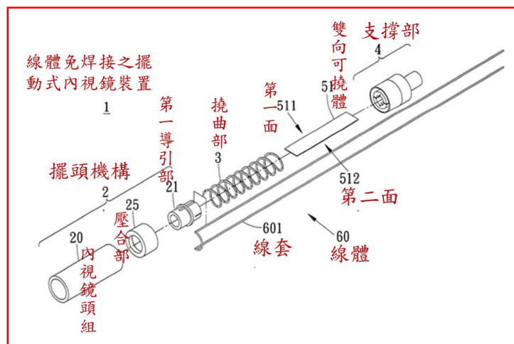
第 1 圖為系爭專利線體免焊接之擺動式內視鏡裝置之分解示意圖
