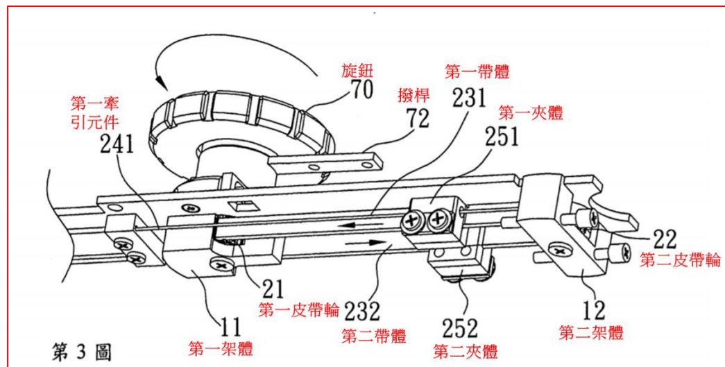
第 3 圖係為可撓管擺頭控制裝置之旋鈕作動示意圖
