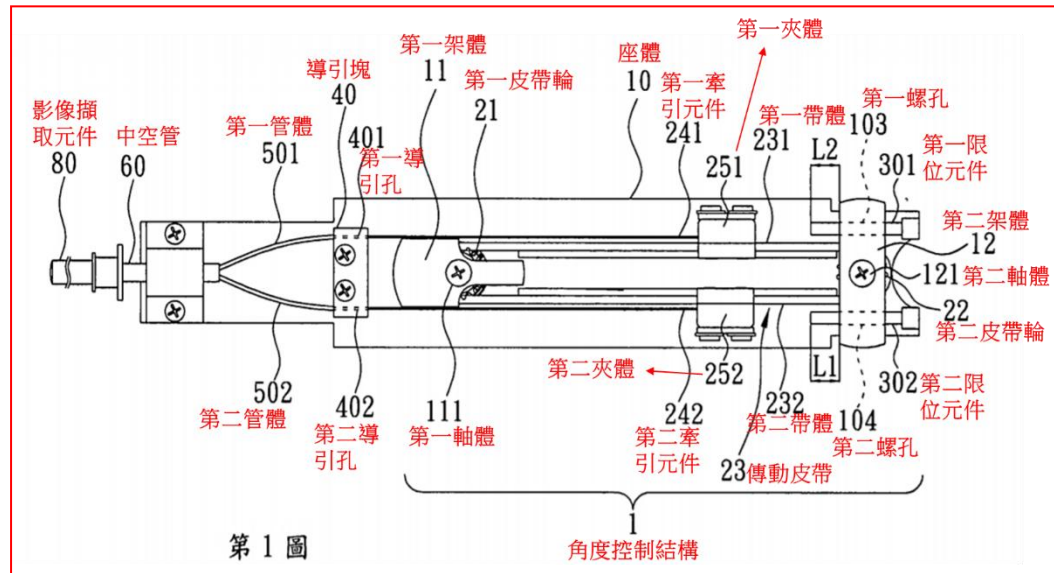
第 1 圖係為可撓管擺頭控制裝置之示意圖
