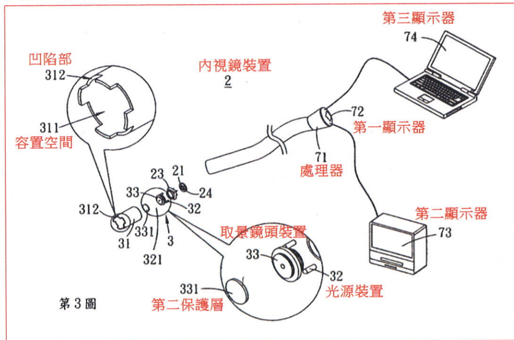
微型攝影裝置之立體結構分解示意圖
