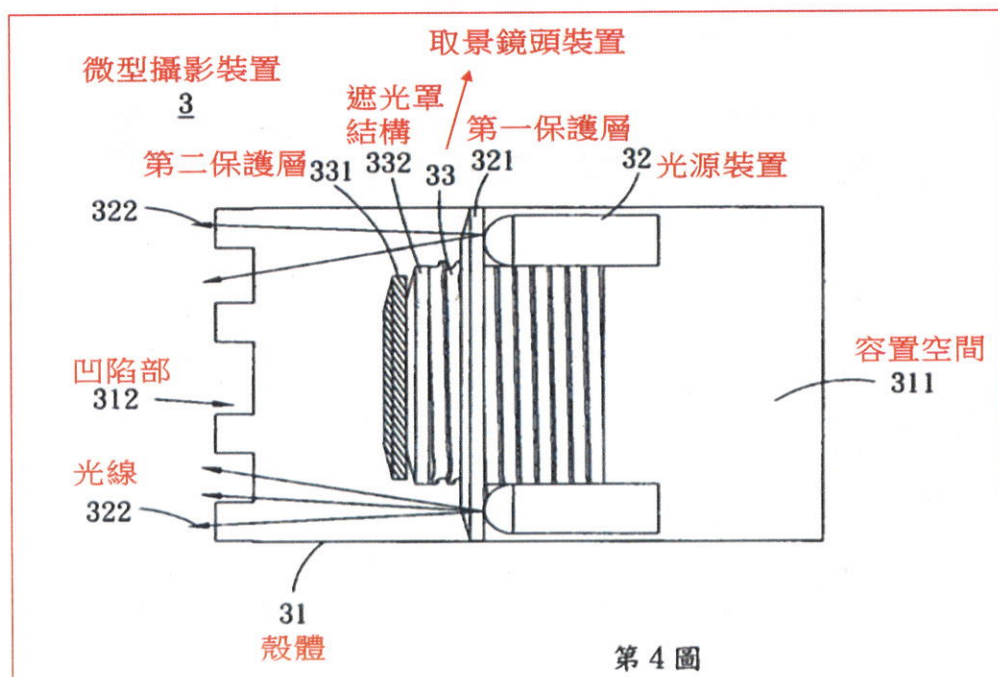
微型攝影裝置之立體結構示意圖
