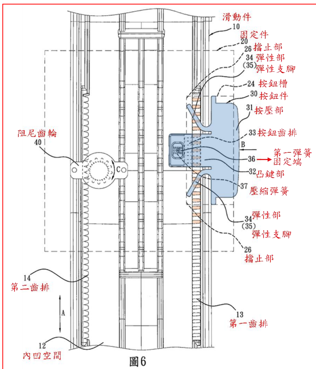
圖 6 係滑動件在被調整移動狀態的平面示意圖
