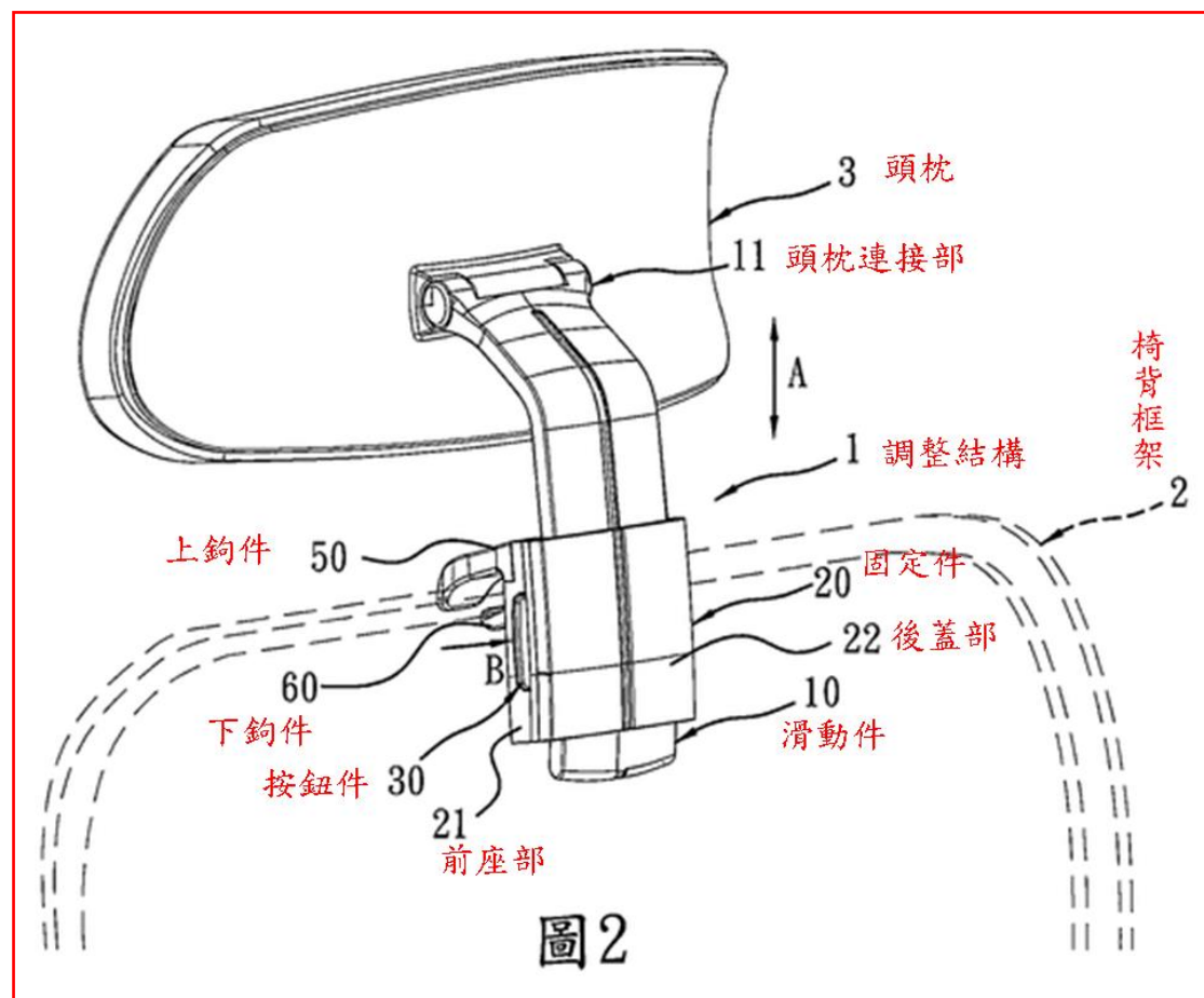
圖 2 係頭枕被調整移動至較高位置的立體組合示意圖
