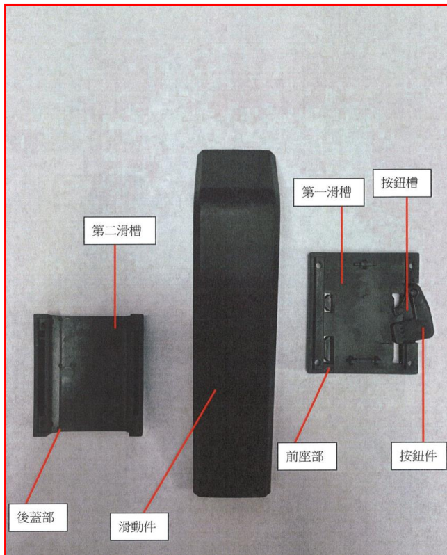
圖 5 系爭產品拆解後外觀圖
