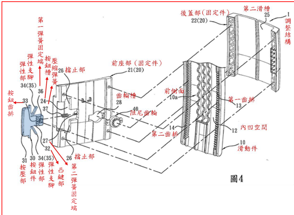
圖 4 係實施例的立體分解示意圖
