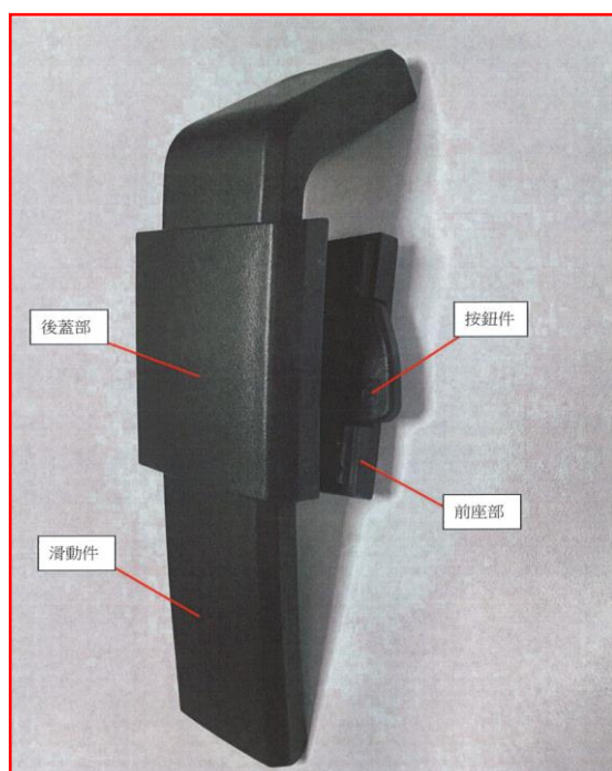
圖 3 系爭產品拆解後外觀圖
