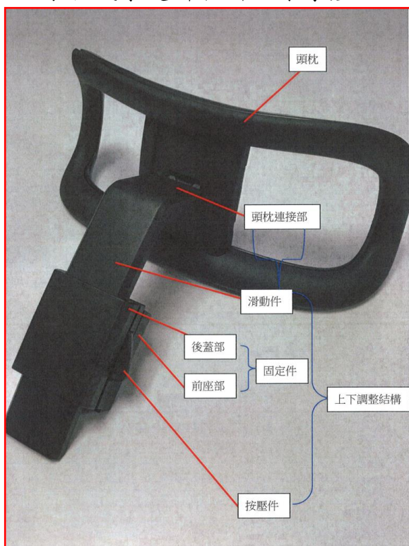
圖 1 系爭產品結合頭枕之外觀圖
