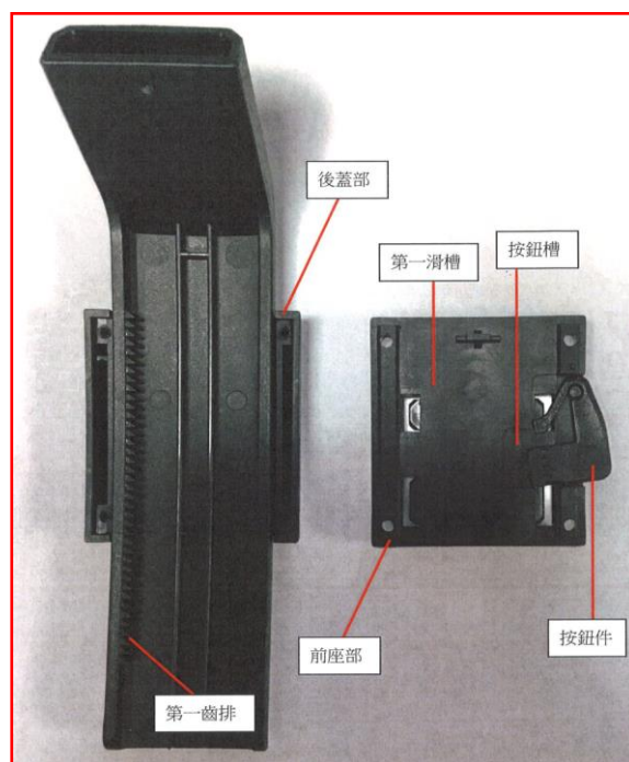
圖 4 系爭產品拆解後外觀圖
