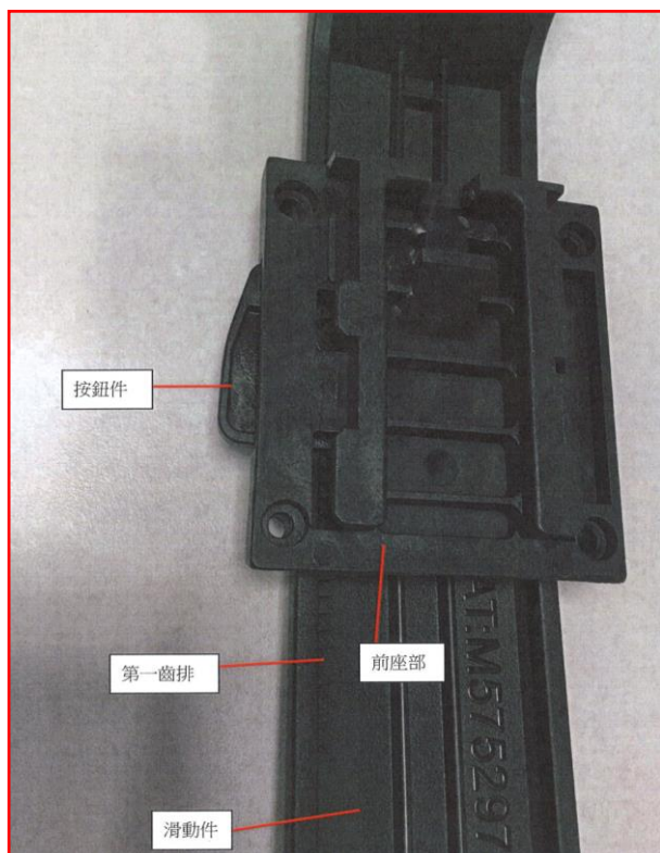
圖 7 系爭產品拆解後外觀圖
